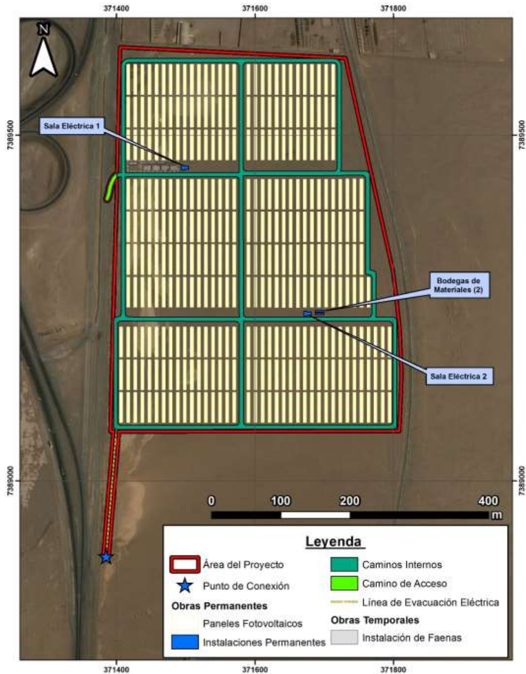
Figura N° 2: Principales obras del Proyecto.
