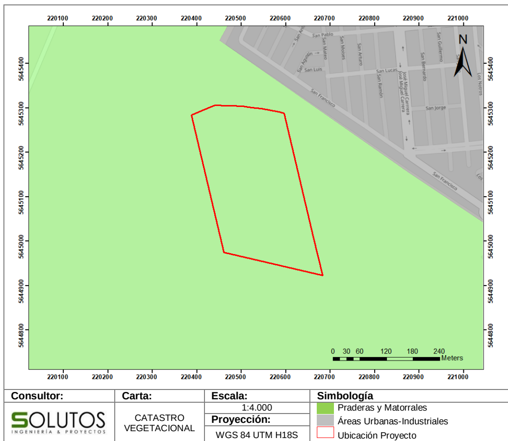
Figura 4. Catastro Vegetacional SIT CONAF 2014
