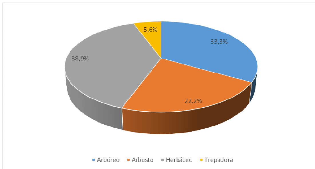
Gráfico 3: División por hábito de crecimiento para el catastro de flora en el área de influencia
