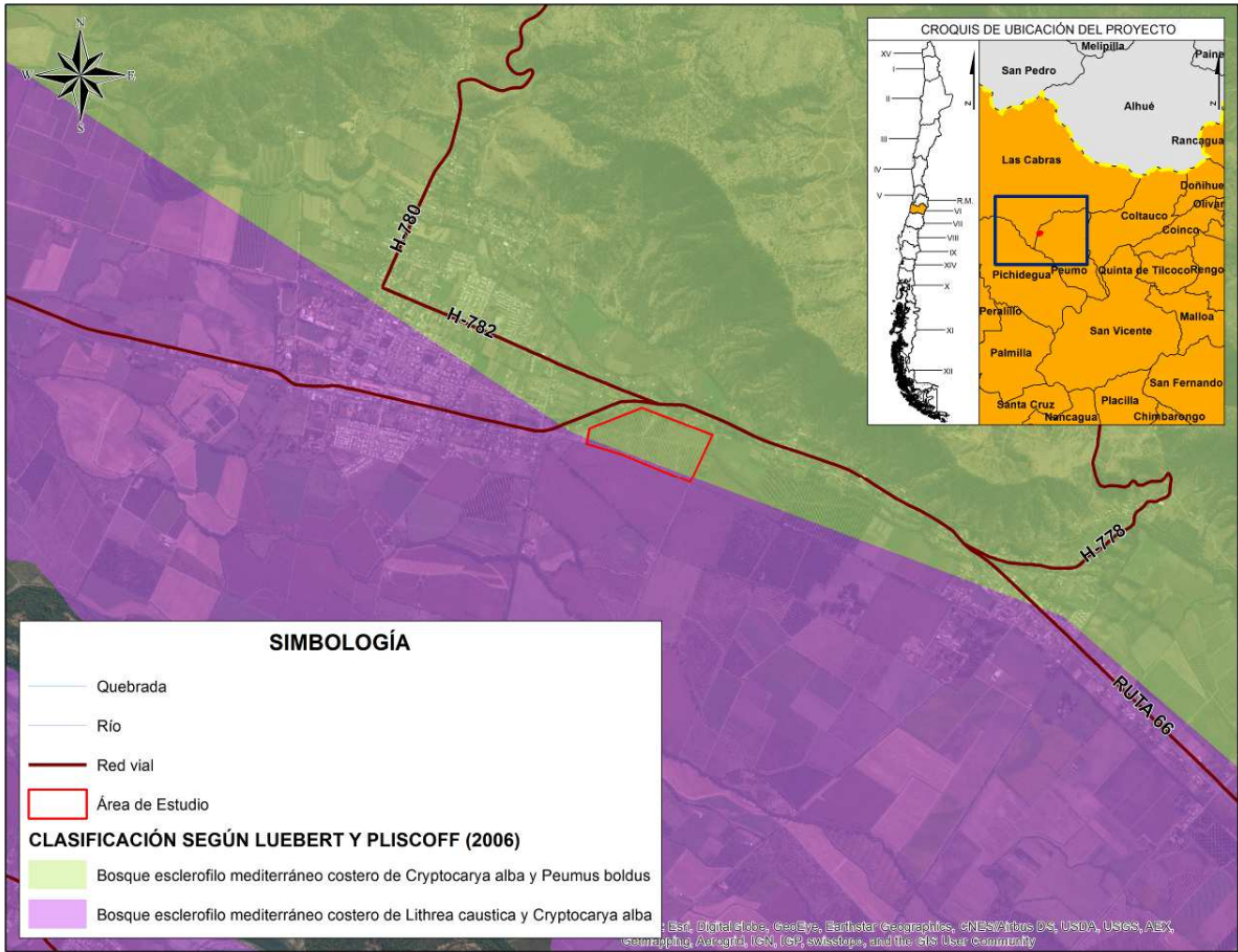
Ilustración 5: Formaciones vegetales del área de estudio de acuerdo a Luebert y Pliscoff (2006)
