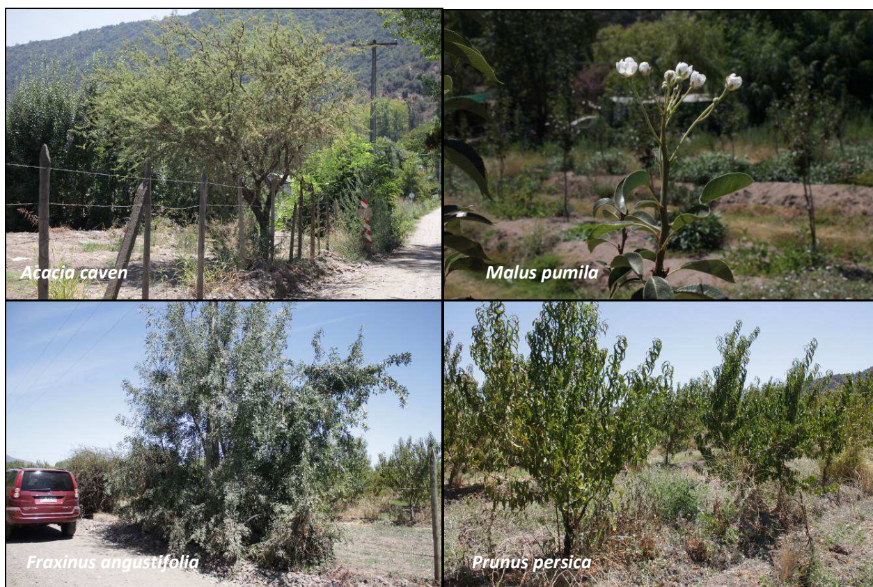
Fotografía 7. Capturas de especies arbóreas identificadas en el área de influencia (Campaña Febrero de 2016)
