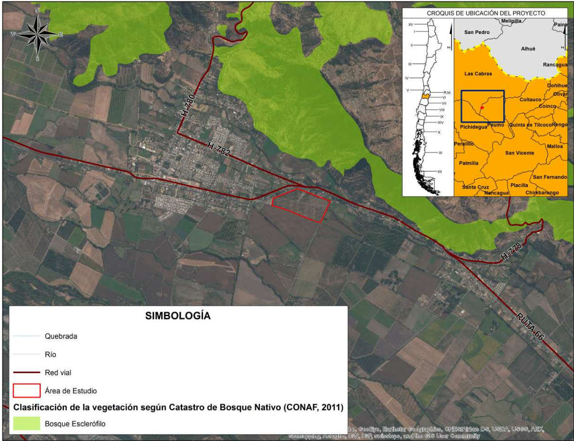
Ilustración 6: Formaciones vegetales del área de estudio de acuerdo a CONAF (2011)
