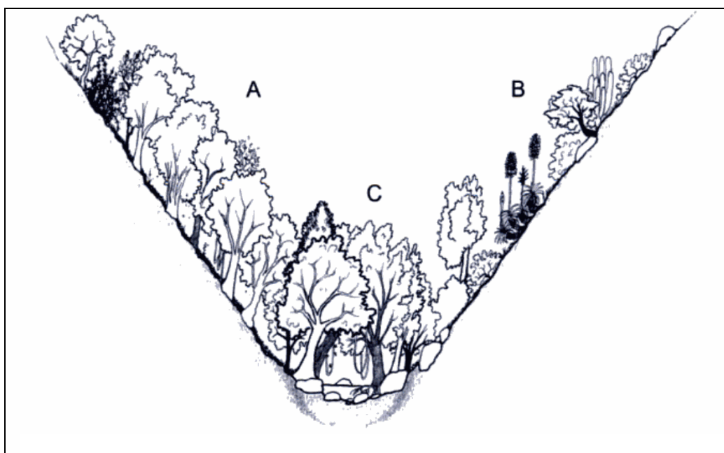
Ilustración 4: Esquema de distribución de la vegetación en el Bosque Esclerófilo Mediterráneo Costero de Cryptocarya alba y Peumus boldus de acuerdo a Luebert y Pliscoff (2006)
