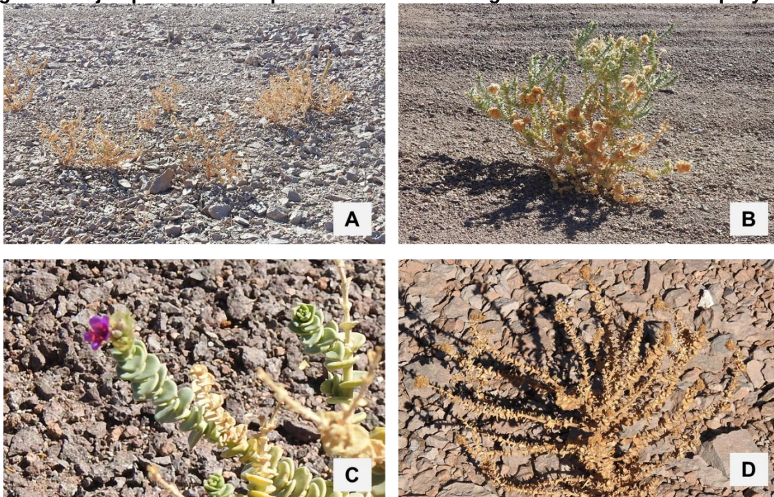
Figura 6-3 Ejemplares de la especie C. salsoloides registrados en el área del proyecto
