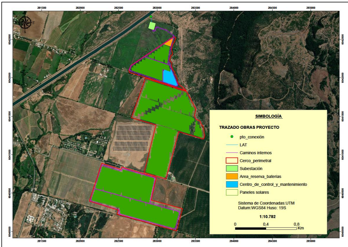
Figura 1. Trazado Obras Proyecto.
