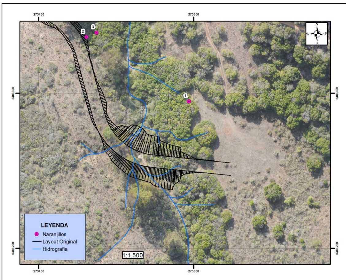
Figura 8. Ubicación de los Naranjillos junto al layout del Camino de acceso a la Planta TAS.
