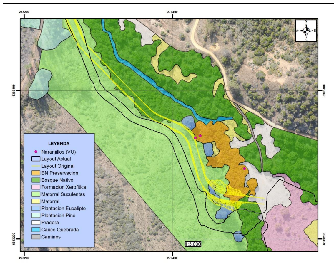
Figura 28. Modificación del layout del camino a la Planta (versión original en amarillo; versión actual, en negro).
