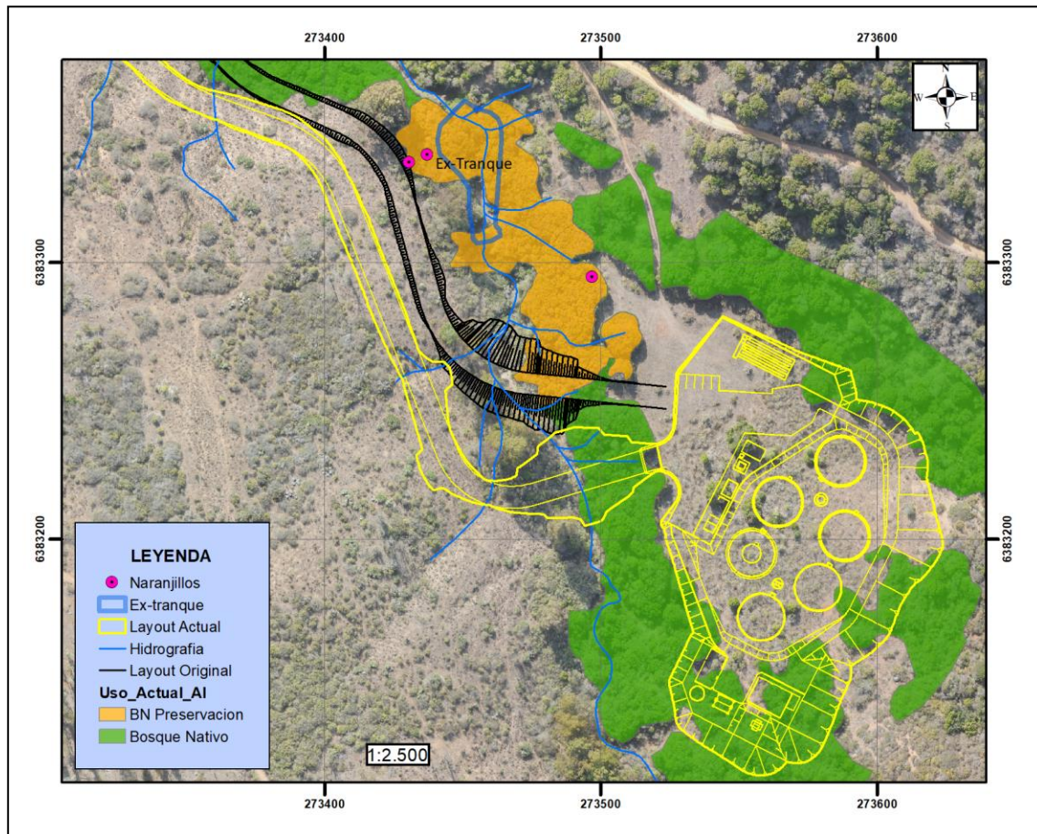
Figura 18. Esquema General de los Layout del Proyecto y su localización respecto el BNP de Naranjillo.
