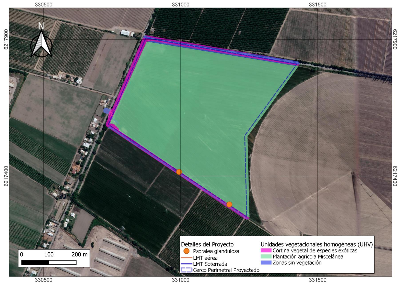
Ilustración 9: Unidades vegetacionales homogéneas
