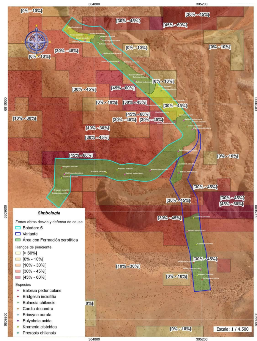
Imagen 7. Rangos de pendientes presentes en el área de proyección obras de manejo de aguas lluvia
