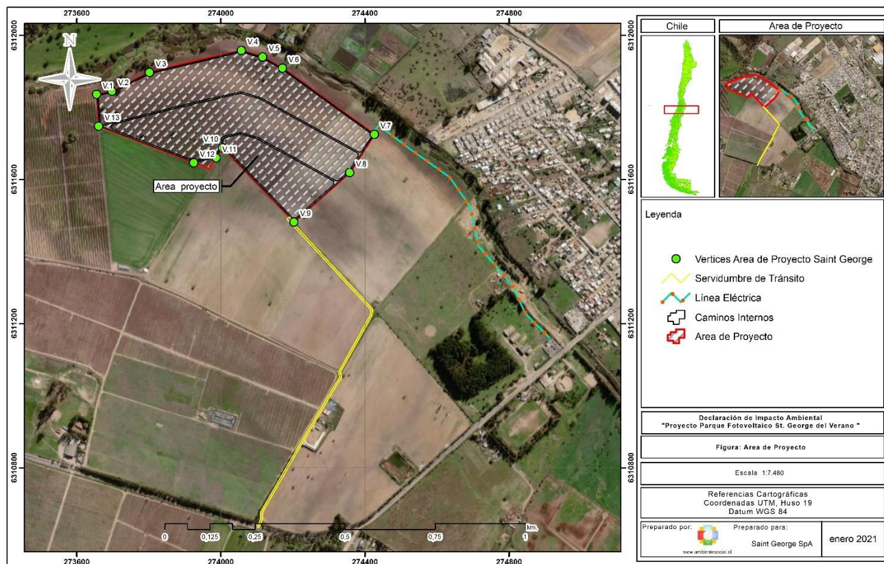
Figura 1. Ubicación geográfica del proyecto “Parque Fotovoltaico Saint George del Verano”
