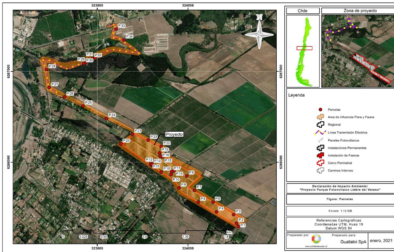
Figura 3. Recorrido en base a parcelas dentro del área de influencia del proyecto "Parque Fotovoltaico Liebre del verano".
