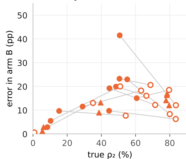
GPT + Python
