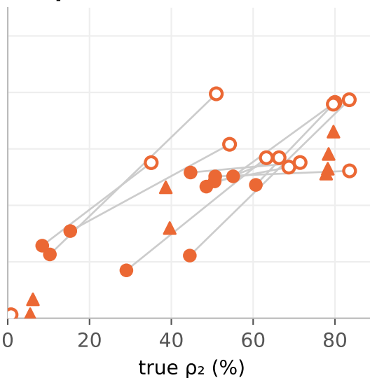
DeepSeek
