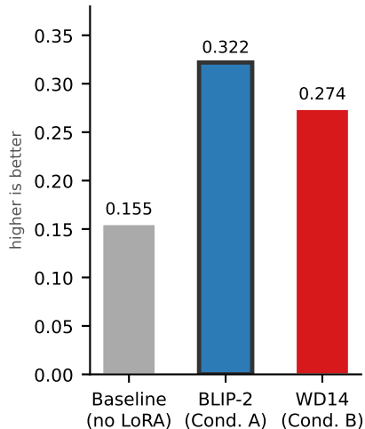
DINOv2 sim.
