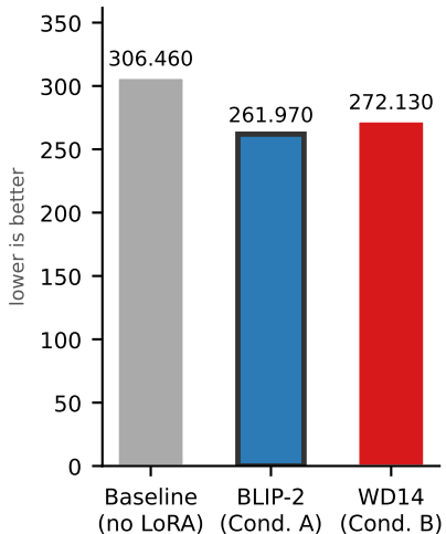
FID
