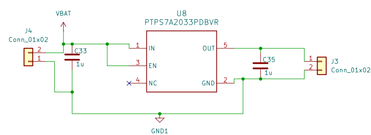
Régulateur LDO (TPS7A20)
