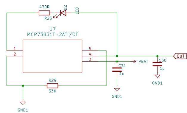
Chargeur Li-Ion (MCP73831)
