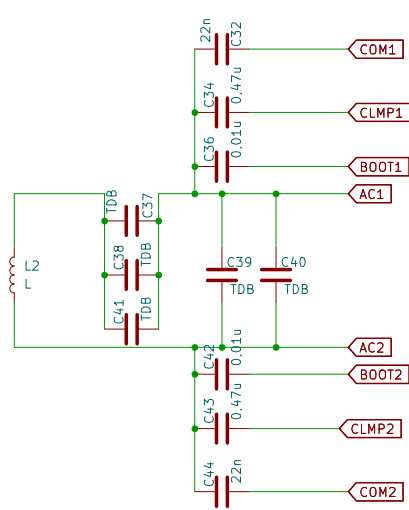
Circuit Résonant & Analogique
