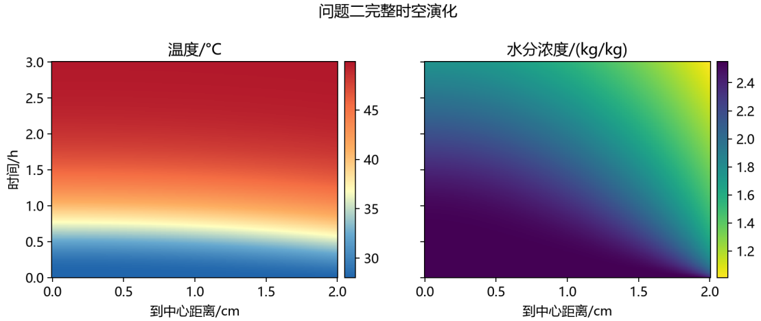
图 7: 问题 2 前 3 h 温度场与水分场的二维时空全景演化热力图
