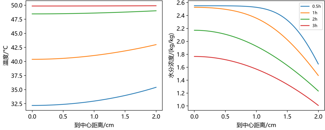
图 6: 问题 2 在代表时刻的径向温度与水分浓度分布剖面
