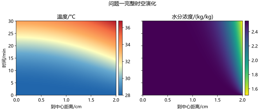
图 5: 问题 1 前 30 min 温度场与水分场的二维时空全景演化热力图
