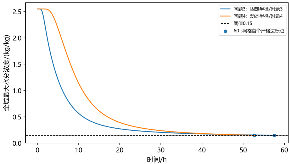
图 8: 问题 3 与问题 4 全域最大水分浓度随时间演化曲线及 60 s 达标点定位
