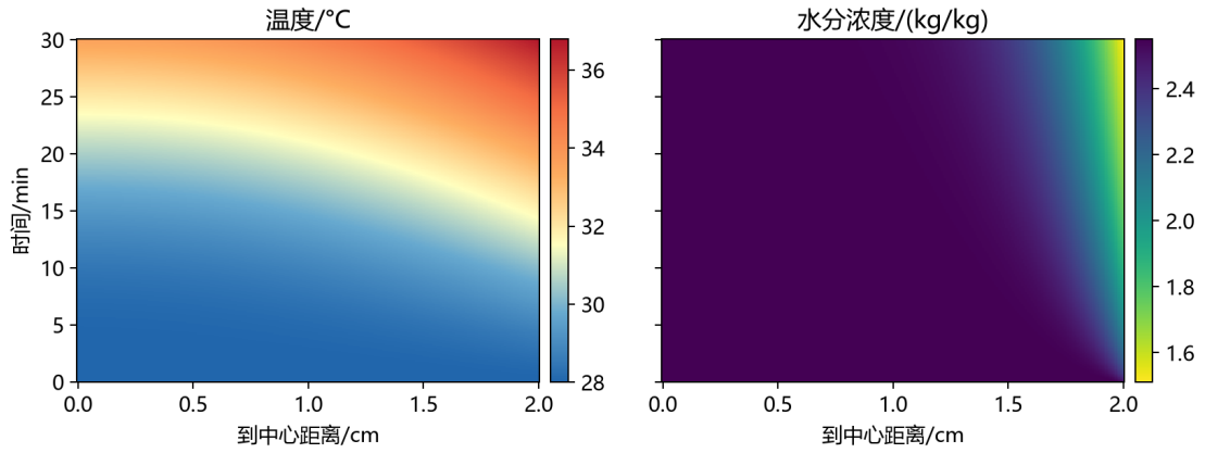
图 4: 问题 1 前 30 min 温度场与水分场的二维时空全景演化热力图
