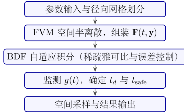
图 2: FVM-BDF 数值求解流程
