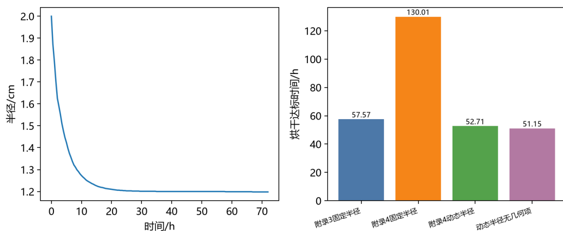
图 13: 附件 2 药材半径实测变化曲线（左）与不同模型烘干达标时间对比柱状图（右）
