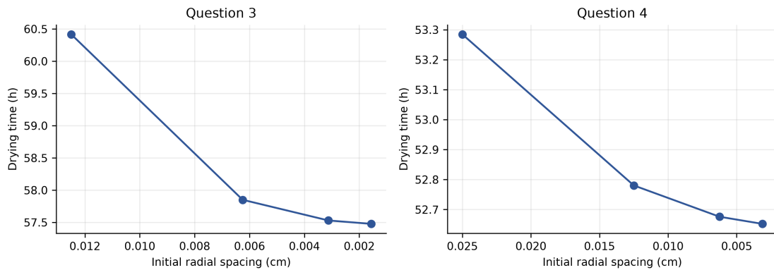
图 11: 问题 3 与问题 4 的径向网格收敛性分析
