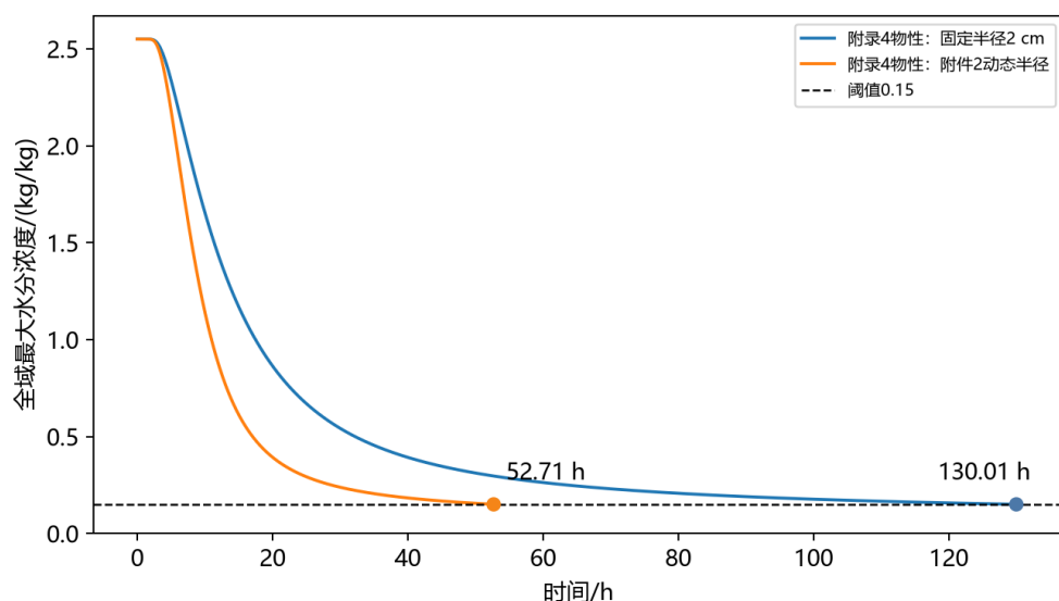
图 12: 附录 4 物性下固定半径与动态收缩的干燥历程对比
