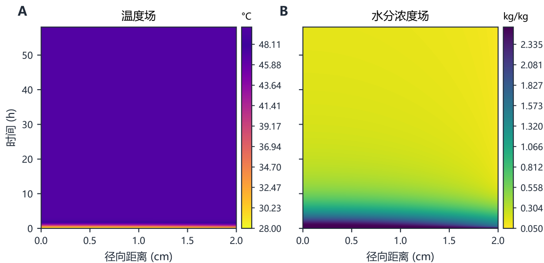
图 9: 问题 3 直至达标后 0.5 h 的温度场与水分场二维时空演化热力图
