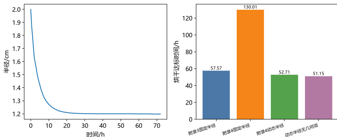
图 10: 附件 2 药材半径实测变化曲线（左）与不同模型烘干达标时间对比柱状图（右）
