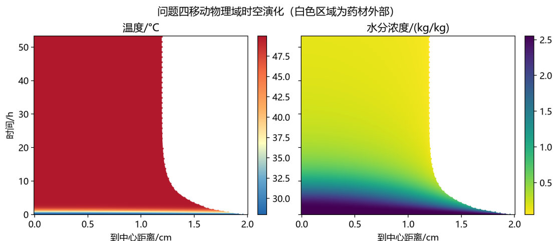
图 11: 问题 4 移动物理域温湿场时空演化热力图（白色区域为药材收缩后的外部空间）
