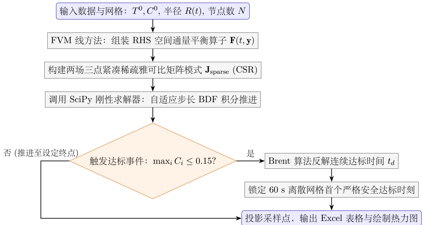
图 2: 基于线方法 FVM 空间半离散与稀疏雅可比自适应 BDF 的统一数值求解流程
