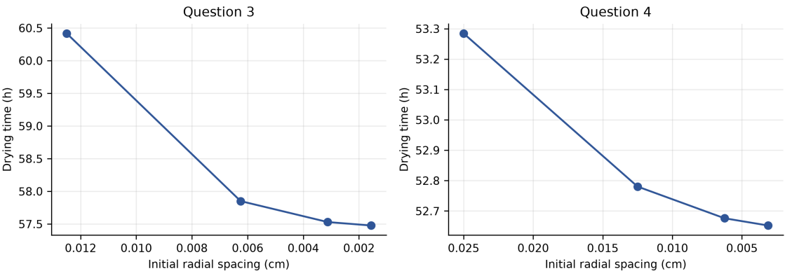
图 4: 问题 3、4 的空间网格收敛
