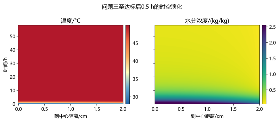
图 9: 问题 3 直至关达标后 0.5 h 的温度场与水分场二维时空演化热力图
