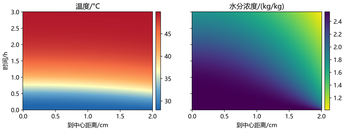
图 7: 问题 2 前 3 h 温度场与水分浓度场的二维时空分布
