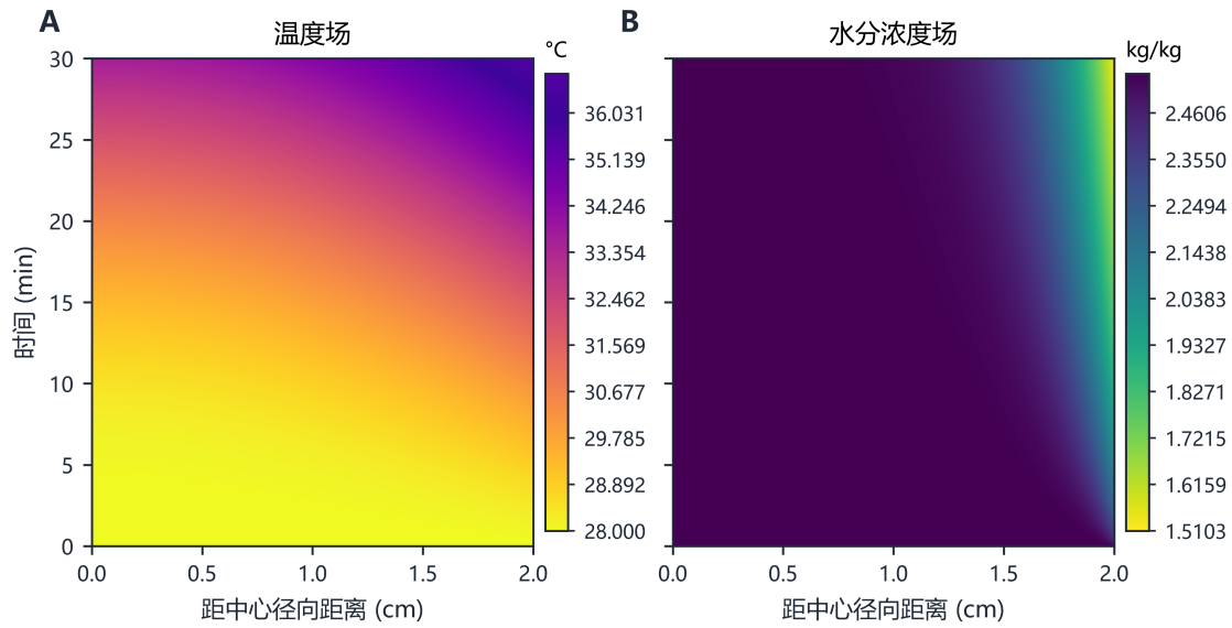
图 5: 问题 1 前 30 min 温度场与水分浓度场的二维时空演化热力图
