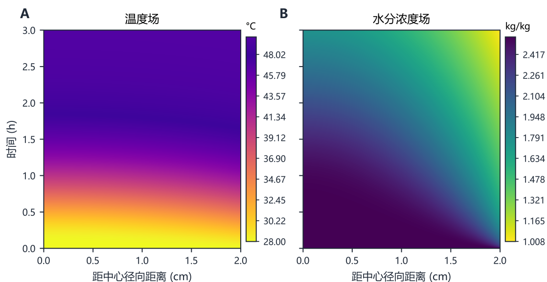
图 7: 问题 2 前 3 h 温度场与水分浓度场的二维时空分布
