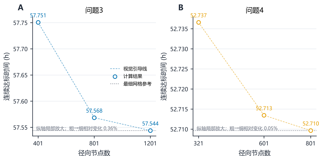
图 11: 问题 3 与问题 4 的径向网格收敛性分析
