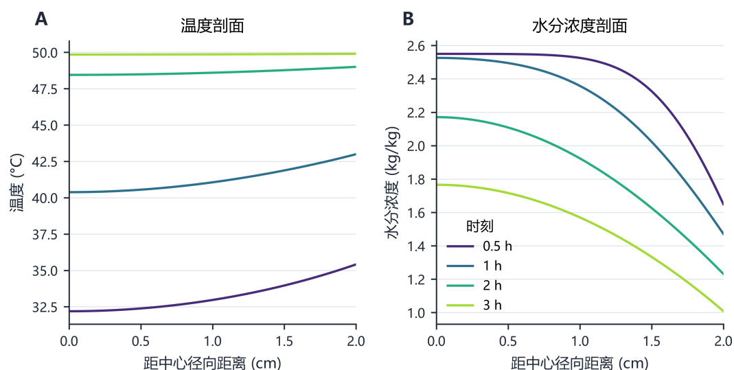
图 6: 问题 2 在代表时刻的径向温度与水分浓度分布
