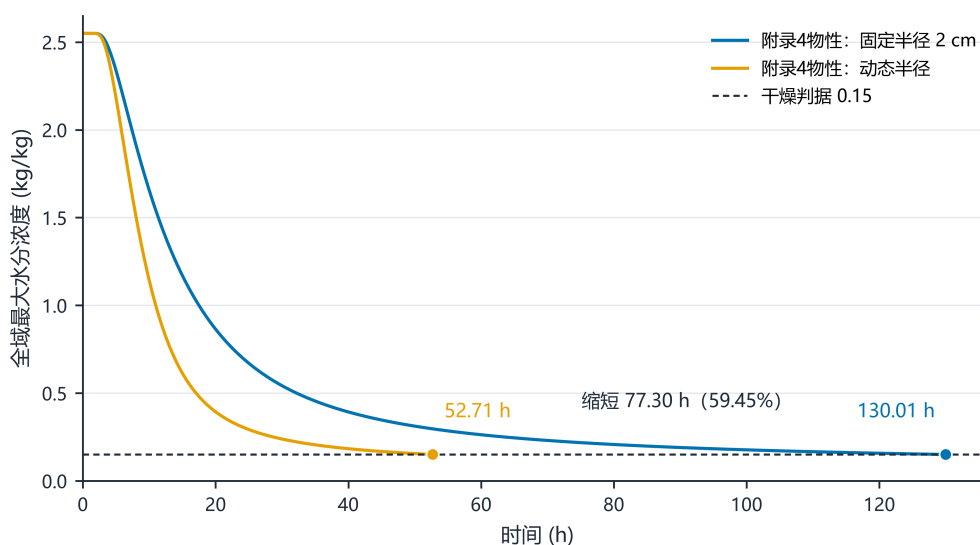
图 12: 附录 4 物性下固定半径与动态收缩的干燥历程对比
