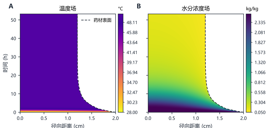
图 10: 问题 4 移动物理域温湿场时空演化热力图（白色区域为药材收缩后的外部空间）
