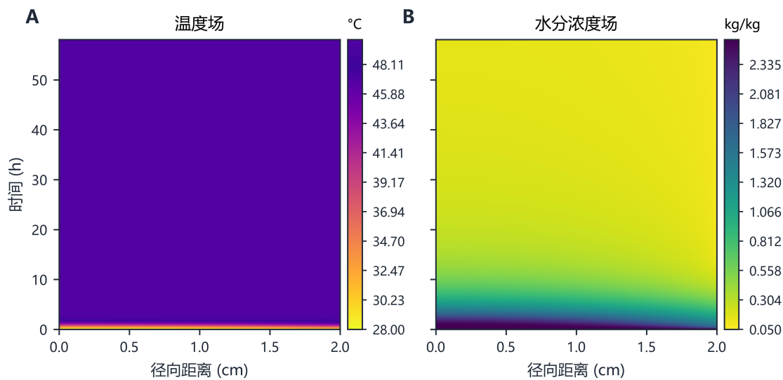
图 9: 问题 3 直至关达标后 0.5 h 的温度场与水分场二维时空演化热力图
