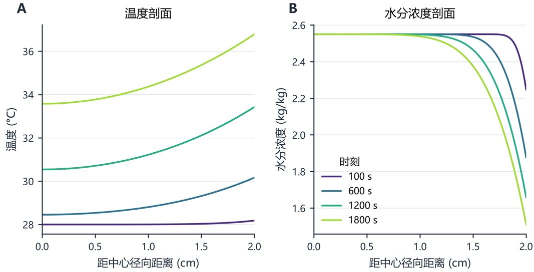
图 4: 问题 1 在不同代表时刻的径向温度与水分浓度分布剖面
