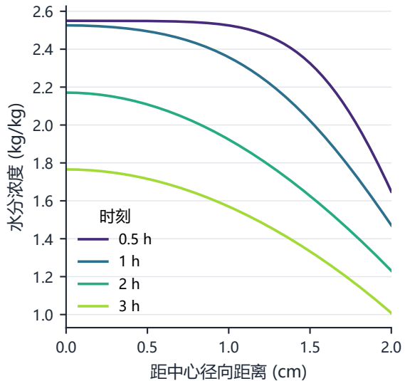
水分浓度剖面
