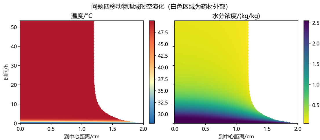
图 10: 问题 4 移动物理域温湿场时空演化热力图（白色区域为药材收缩后的外部空间）
