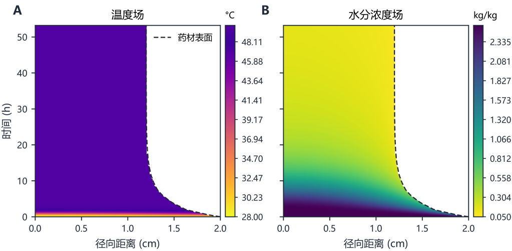
图 10: 问题 4 移动物理域温湿场时空演化热力图（白色区域为药材收缩后的外部空间）
