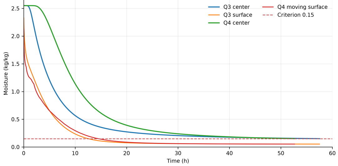
图 4: 问题 3 与问题 4 中心和表面含水率演化
