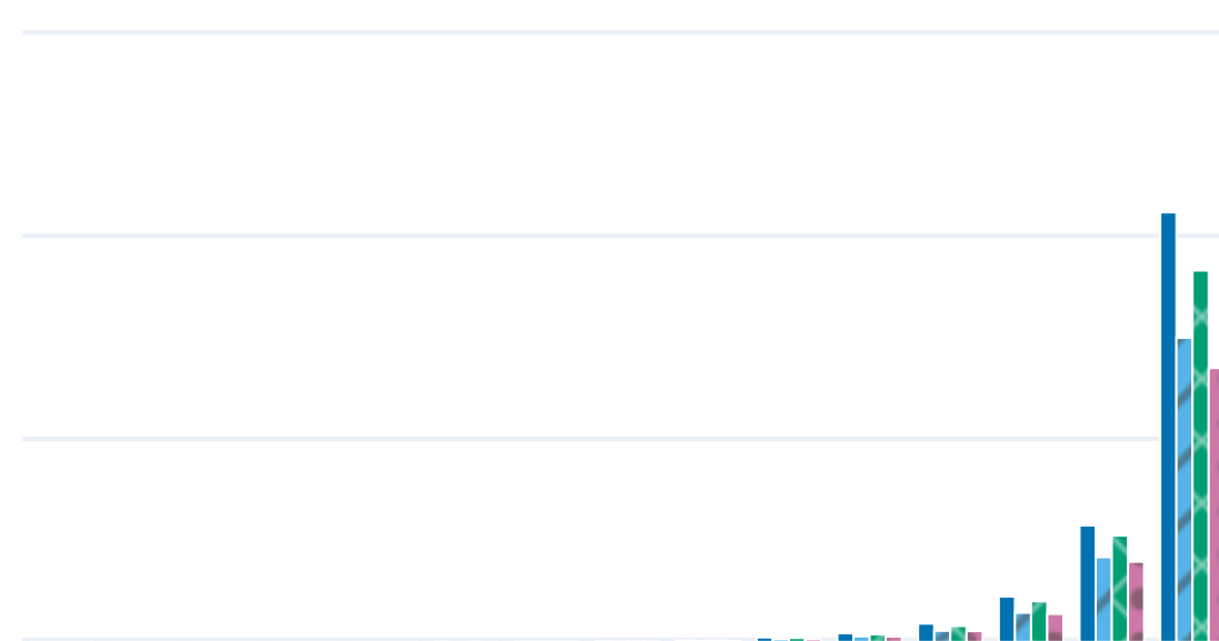
Gzip
