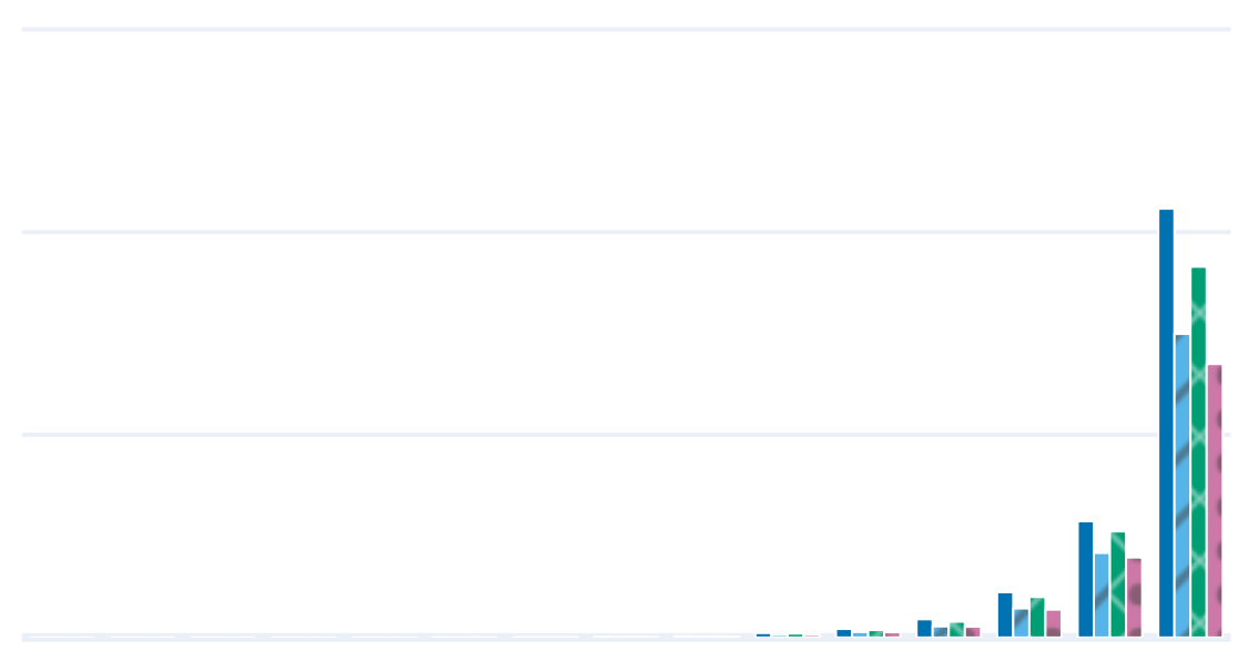
Gzip
