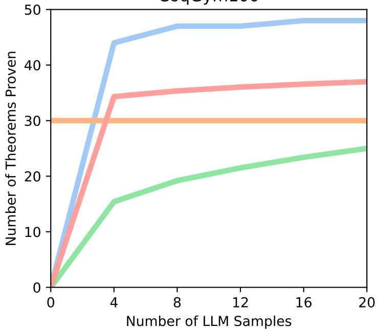
CoqGym100
