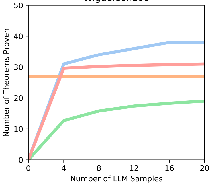
Wigderson100
