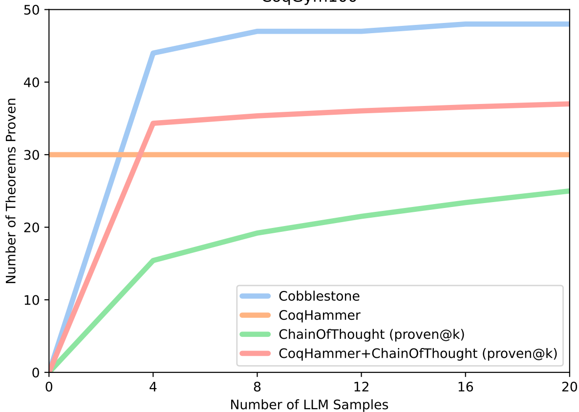
CoqGym100
