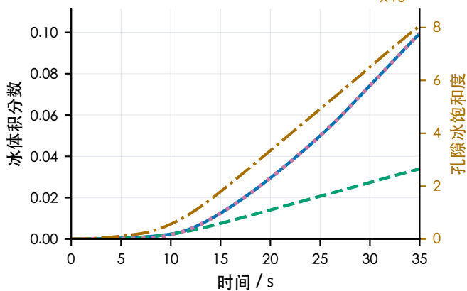
c 含双极板修订 · -20 °C
