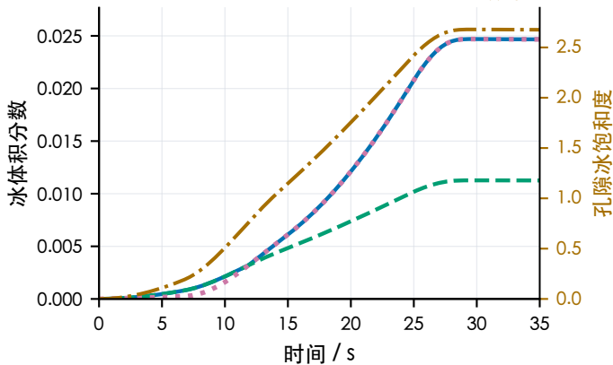
c 含双极板修订 · -20 °C
