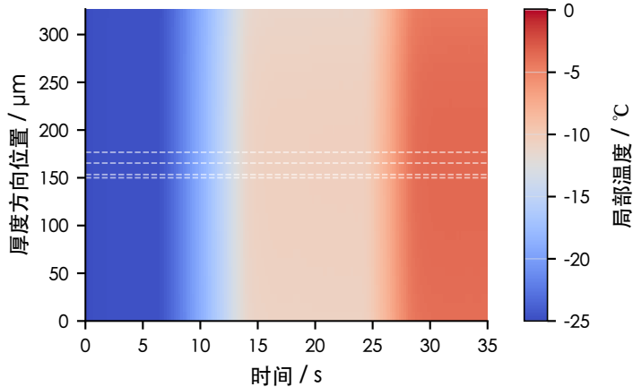
d 初始温度 -25^{\circ}\text{C}
