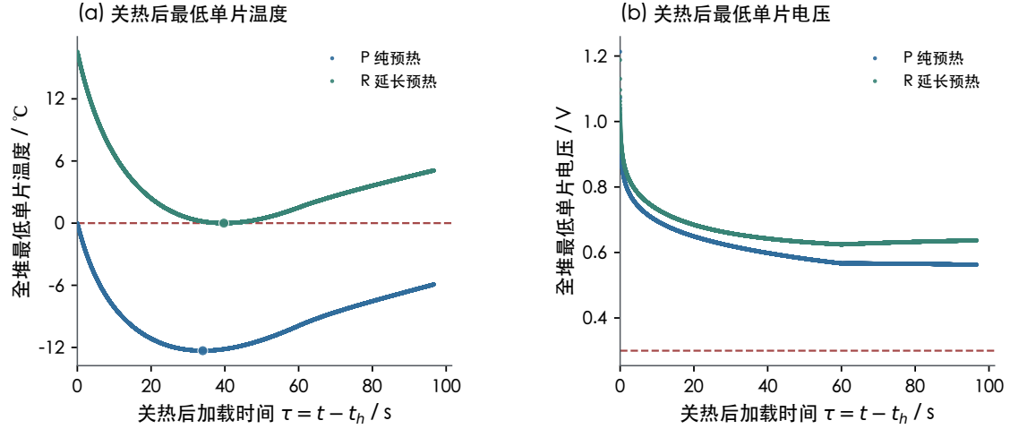
图 6-3 关热后温度回落与延长预热验证图
