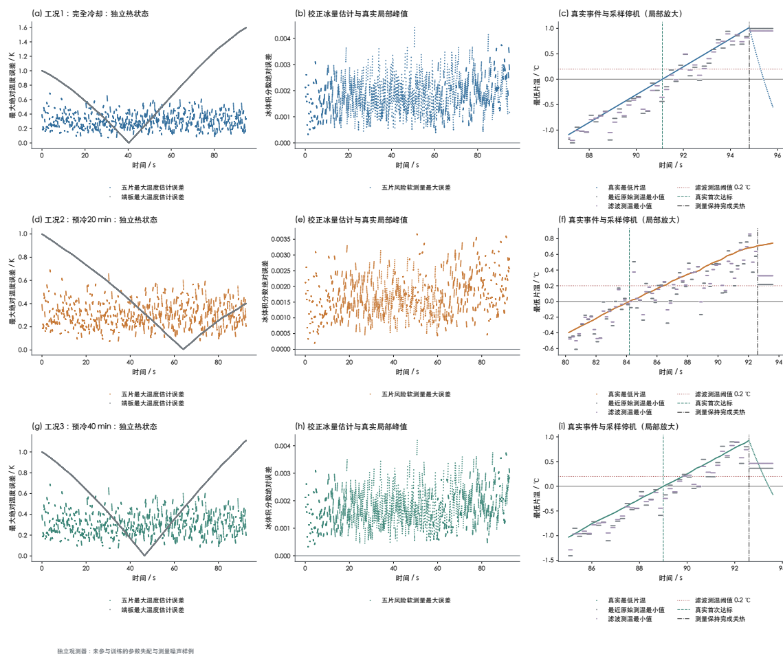
图 7-8 参数失配与测量噪声下的观测误差及停机事件辨析
