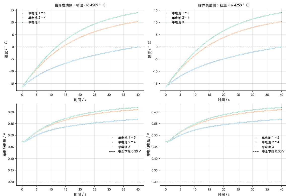
图 5-6 临界初温两侧各单电池温度与电压演化图
