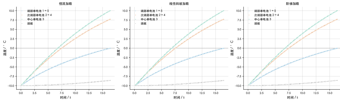
图 5-3 三种加载策略下各单电池与端板温度随时间变化图
