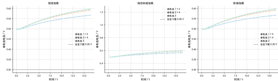
图 5-4 不同加载策略下各单电池电压及安全裕度图
