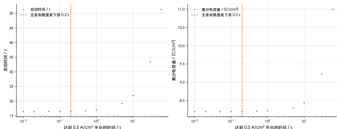
图 5-2 线性升载平台到达时间对启动性能的影响
