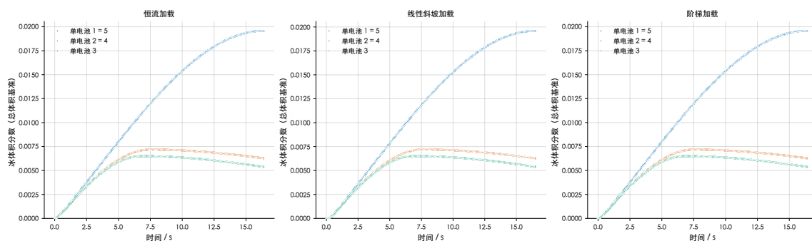
图 5-5 各单电池冰积累程度图
