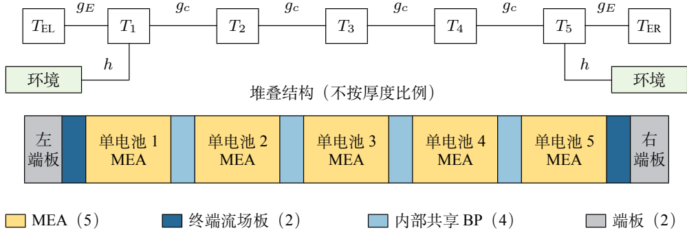
图 5-1 五片电堆结构及热耦合模型示意图
