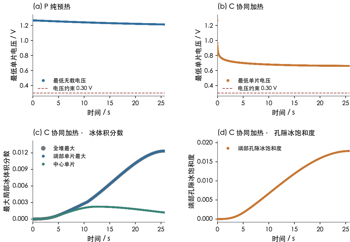
图 6-2 首次启动窗口内两策略电压与协同策略的局部结冰特征
