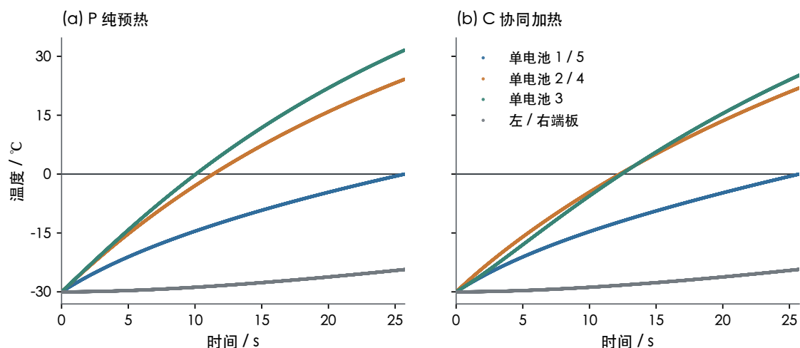
图 6-1 两种主策略温度历程图
