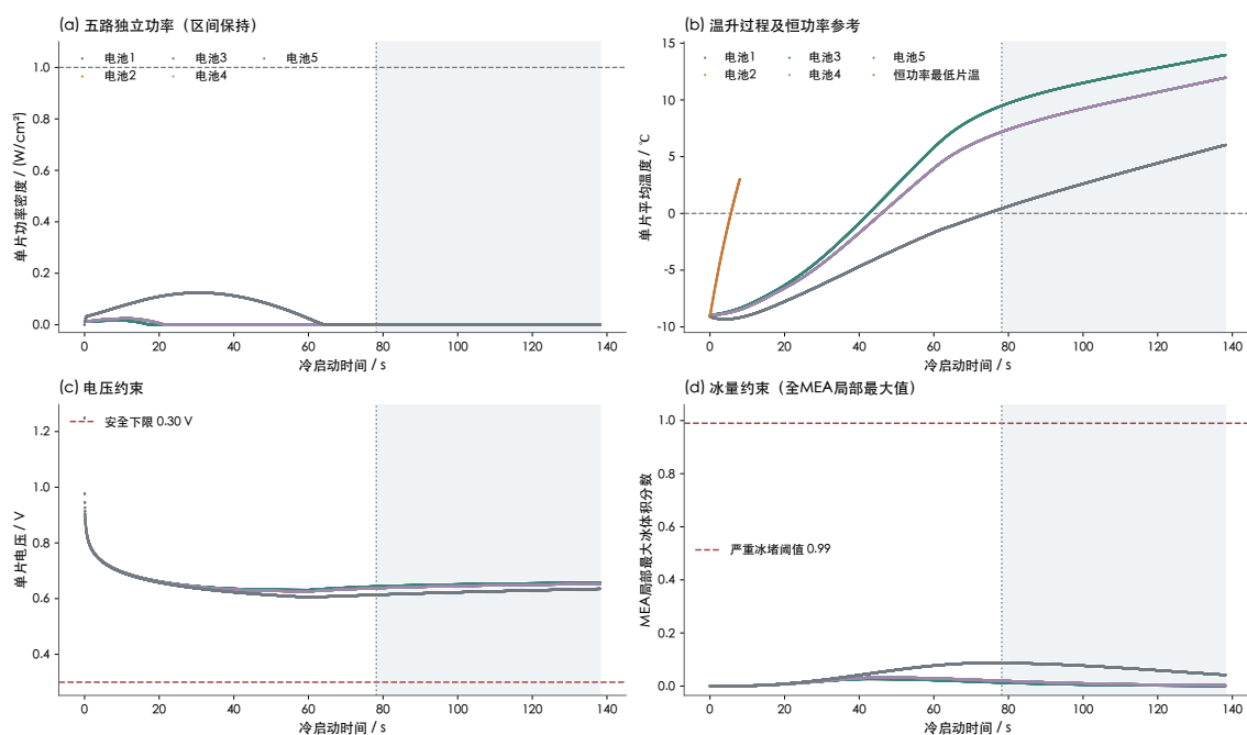
图 7-3 预冷 20 min 工况下推荐动态策略的功率与水热电状态演化
