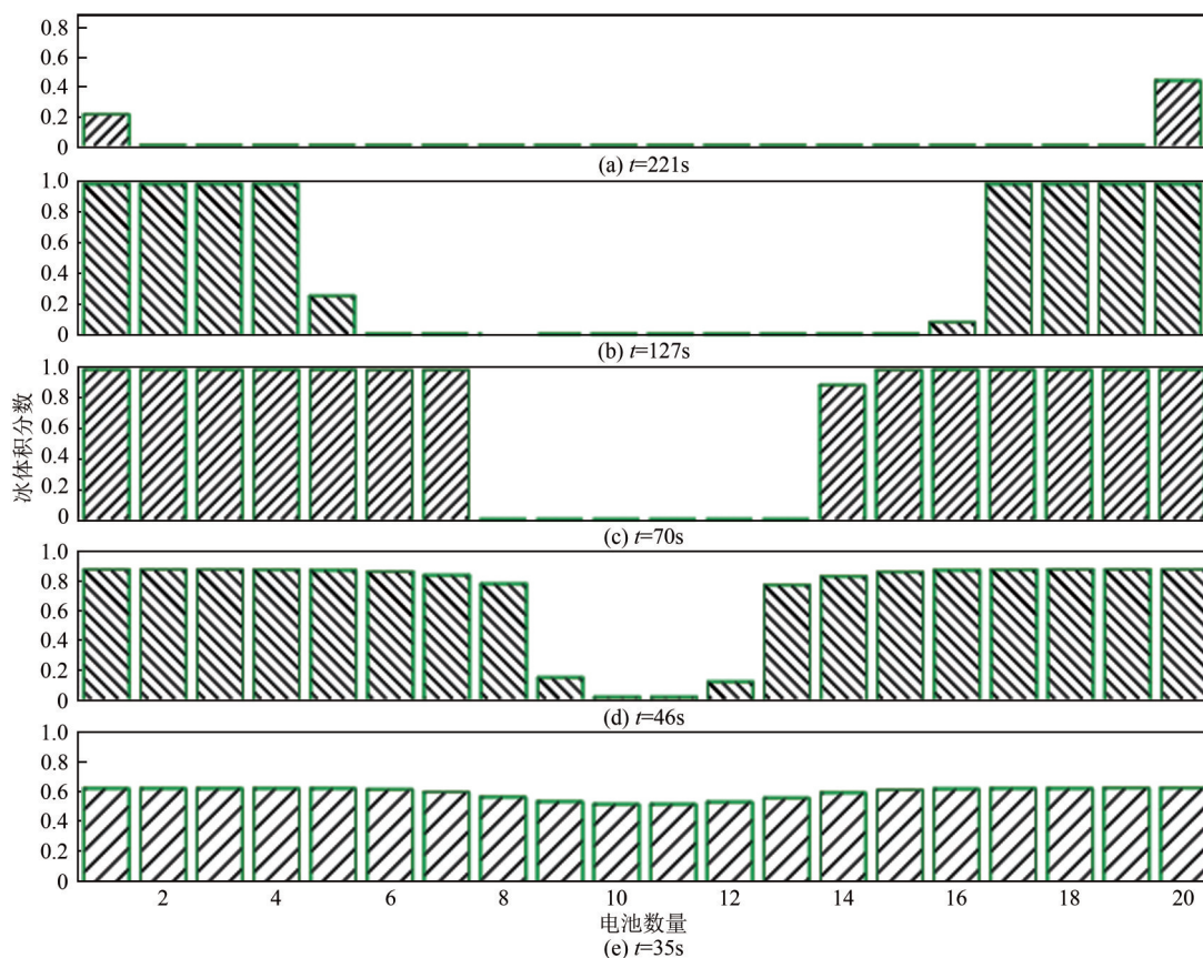
图7 不同电池阴极催化层中的冰体积分数 [30]
