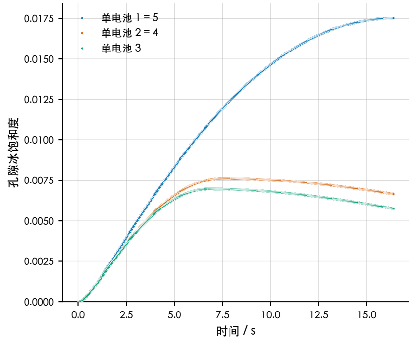
阶梯加载
