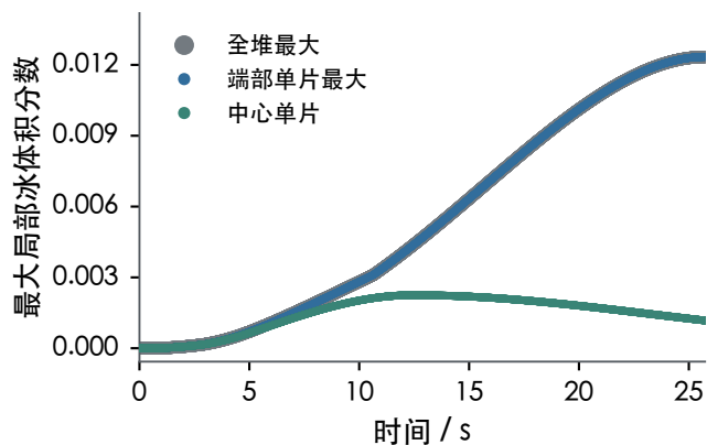
(c) C 协同加热 · 冰体积分数
