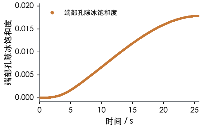
(d) C 协同加热 · 孔隙冰饱和度
