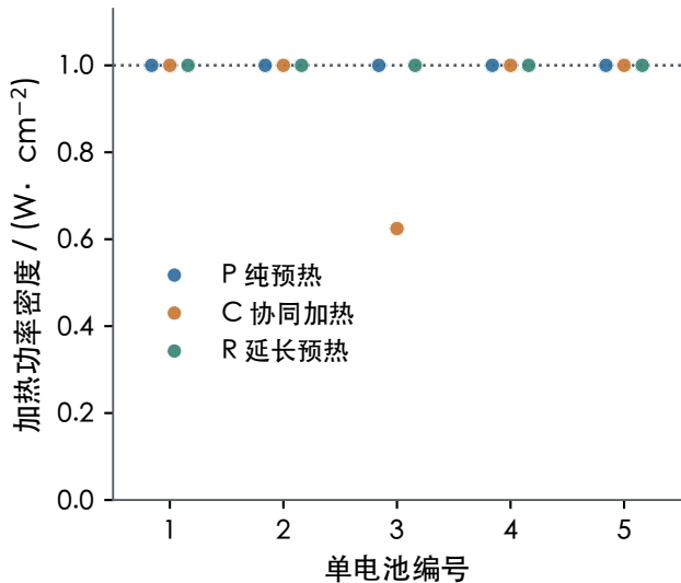
(a) 各片恒定加热功率
