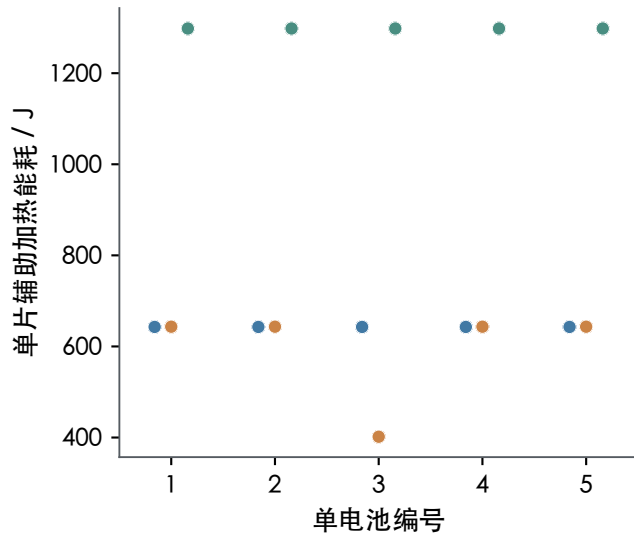
(b) 各片累计辅助能耗
