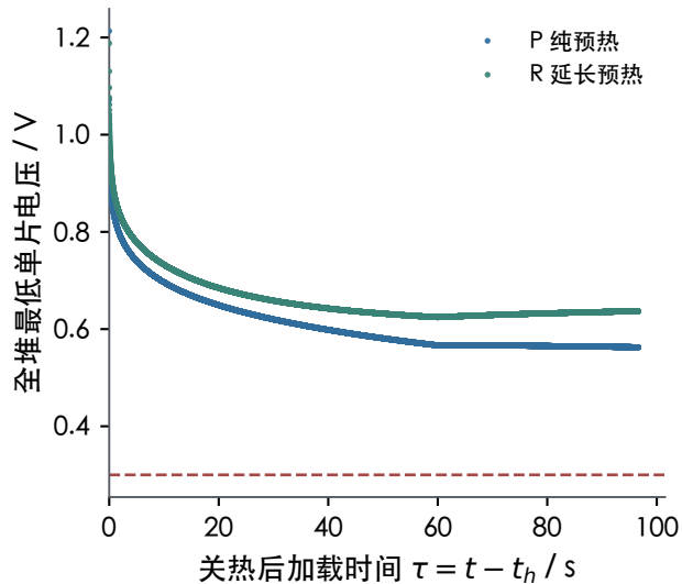
(b) 关热后最低单片电压
