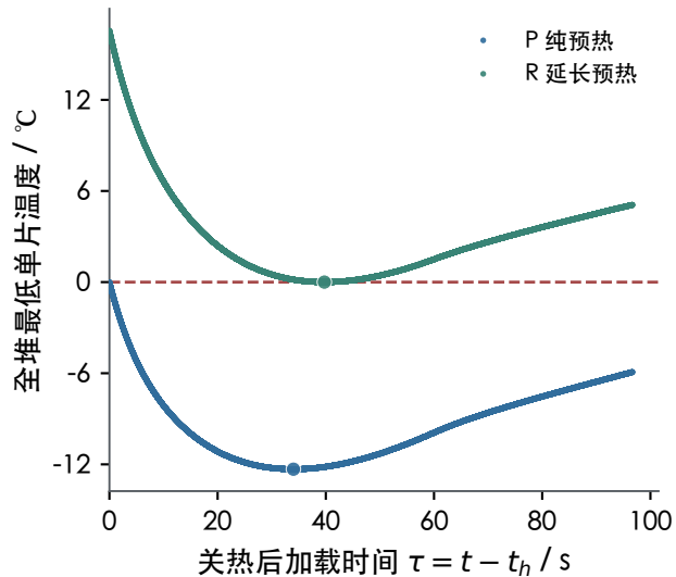
(a) 关热后最低单片温度
