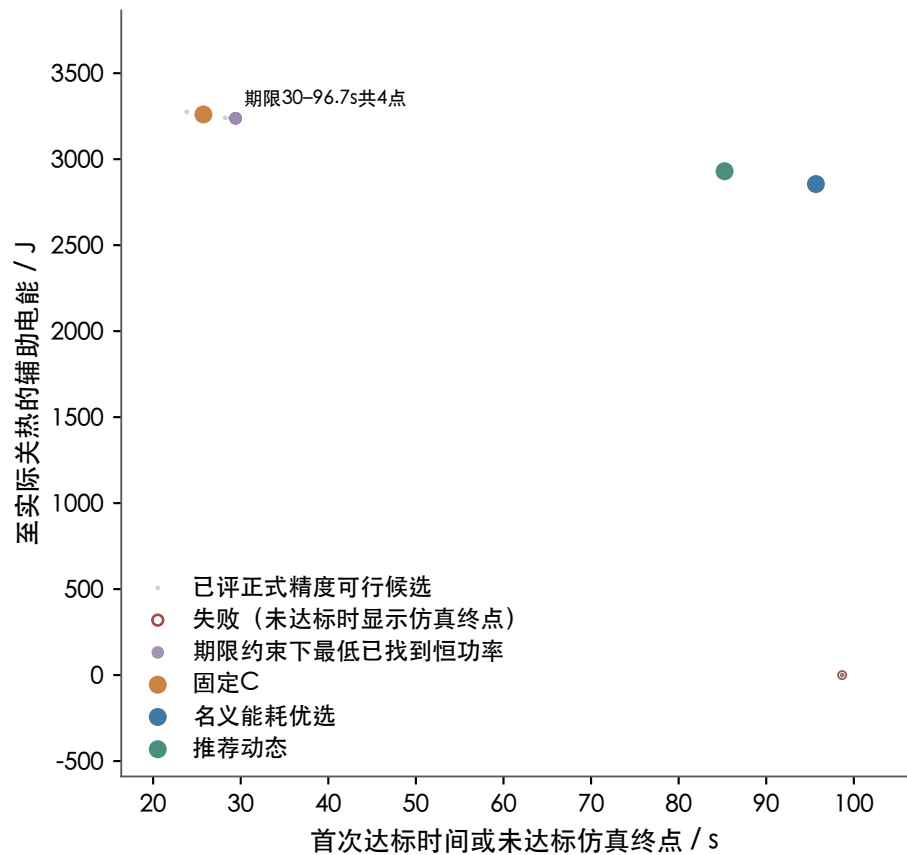
(a) 工况1：完全冷却
