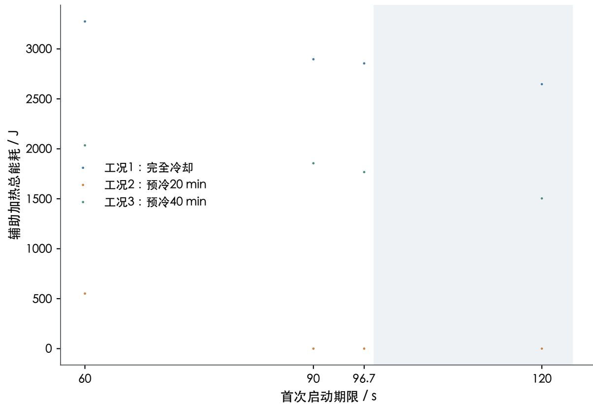
(a) 有限候选集合的最低可行能耗
