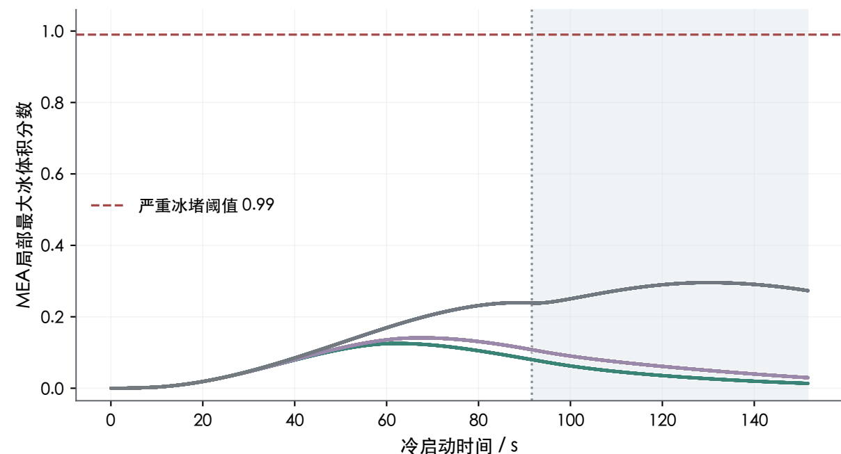
(d) 冰量约束（全MEA局部最大值）
