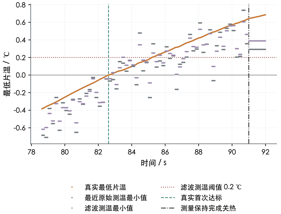
(i) 真实事件与采样停机（局部放大）
