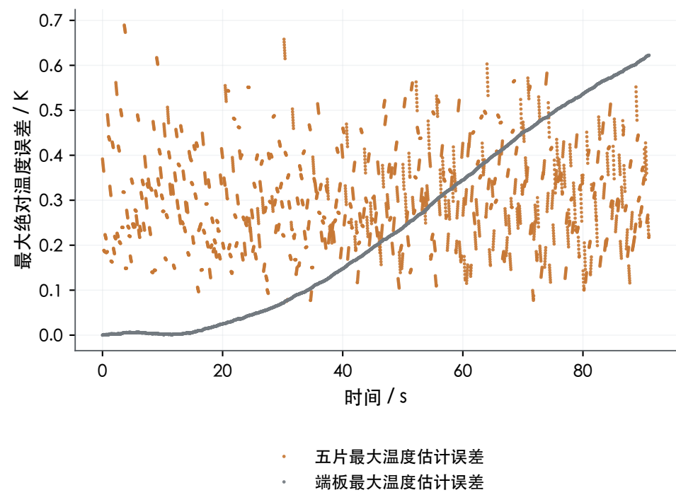
(d) 工况2：预冷20 min：独立热状态
