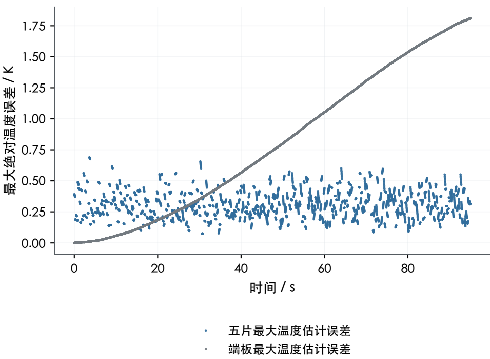
(a) 工况1：完全冷却：独立热状态
