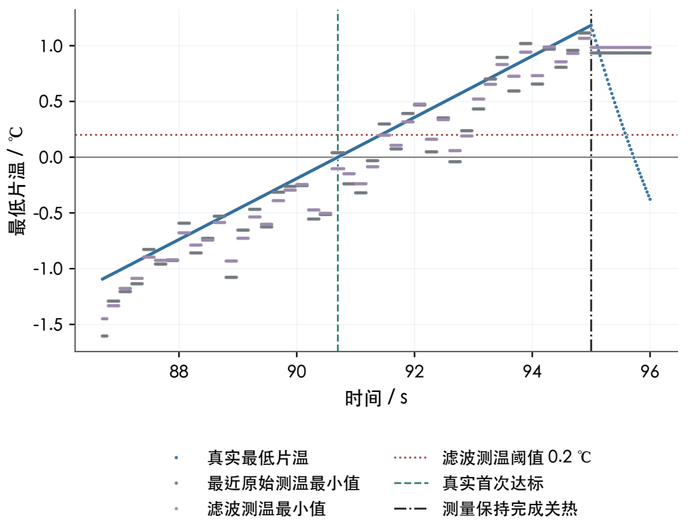
(f) 真实事件与采样停机（局部放大）
