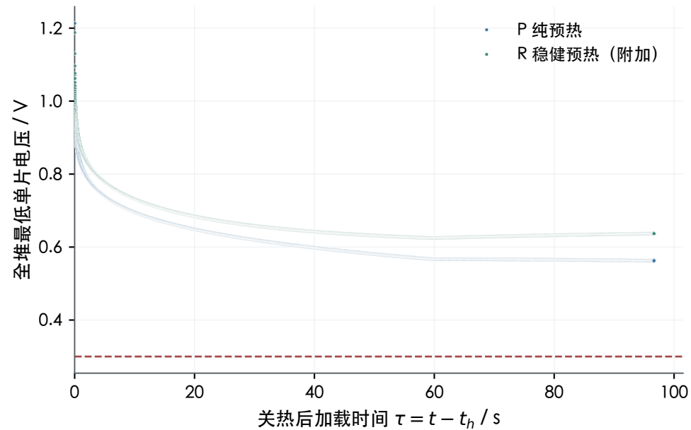
(b) 关热后最低单片电压
