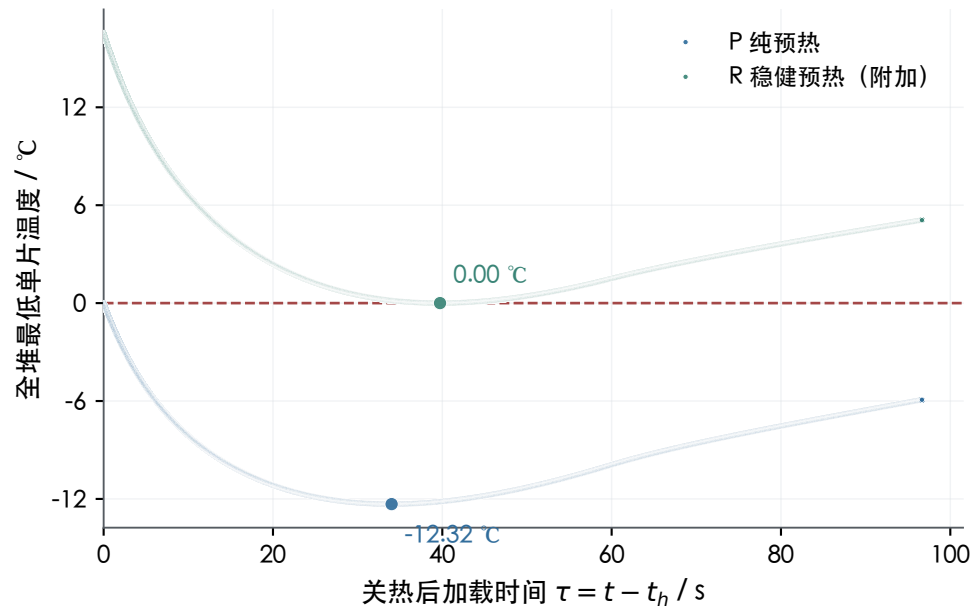
(a) 关热后最低单片温度
