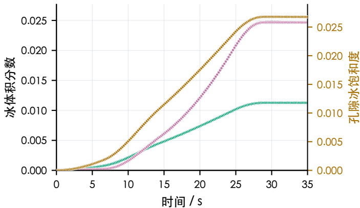
c 含双极板修订 · -20 °C
