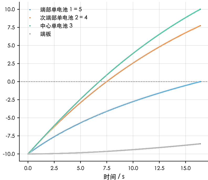
恒流加载
