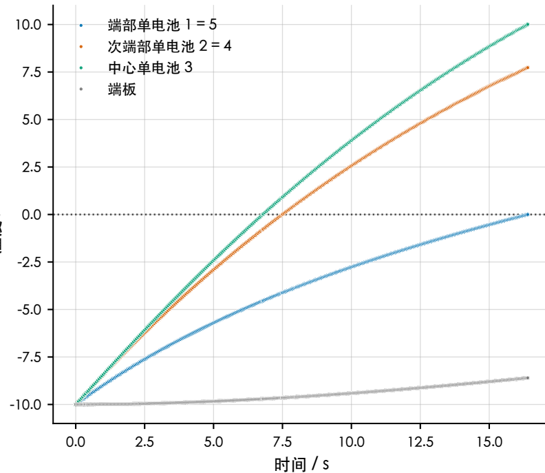
阶梯加载
