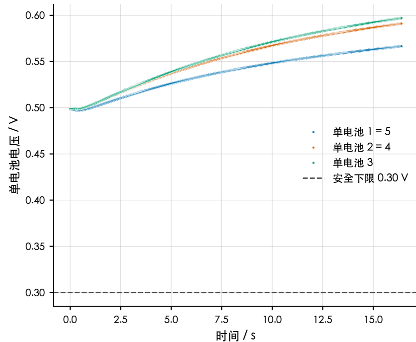
恒流加载
