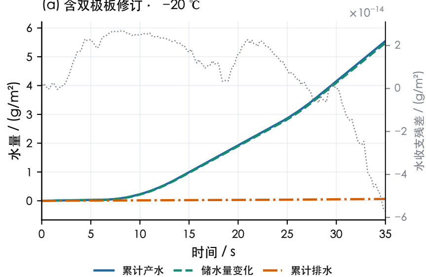
(a) 含双极板修订 · -20 °C
