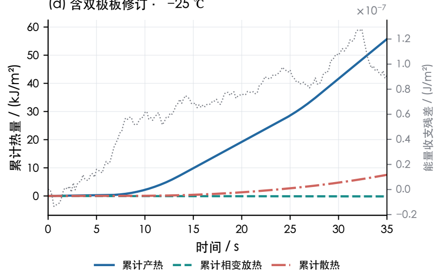
(d) 含双极板修订 · -25 °C
