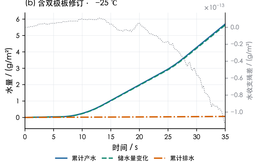
(b) 含双极板修订 · -25 °C
