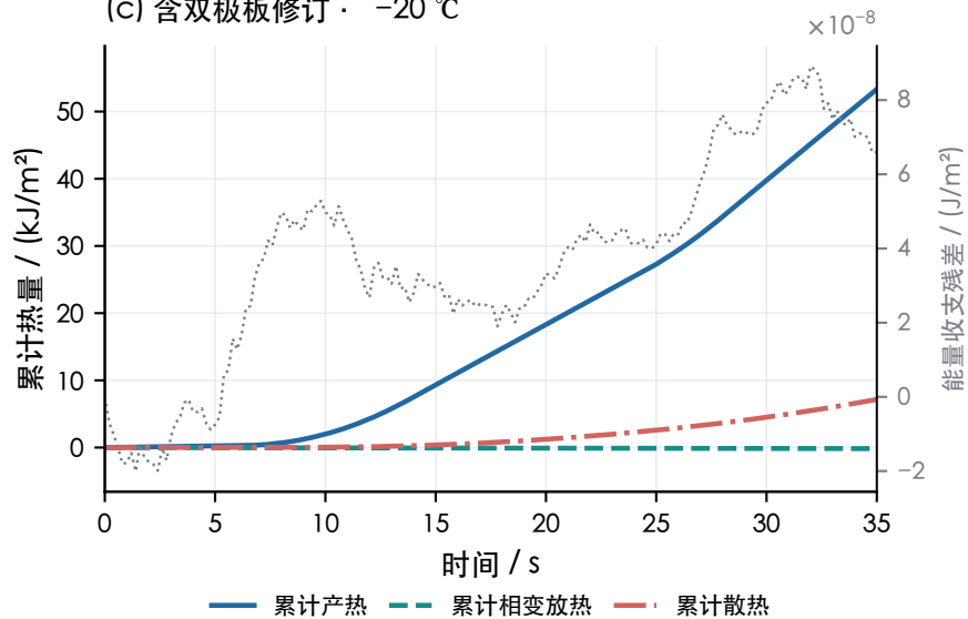
(c) 含双极板修订 · -20 °C
