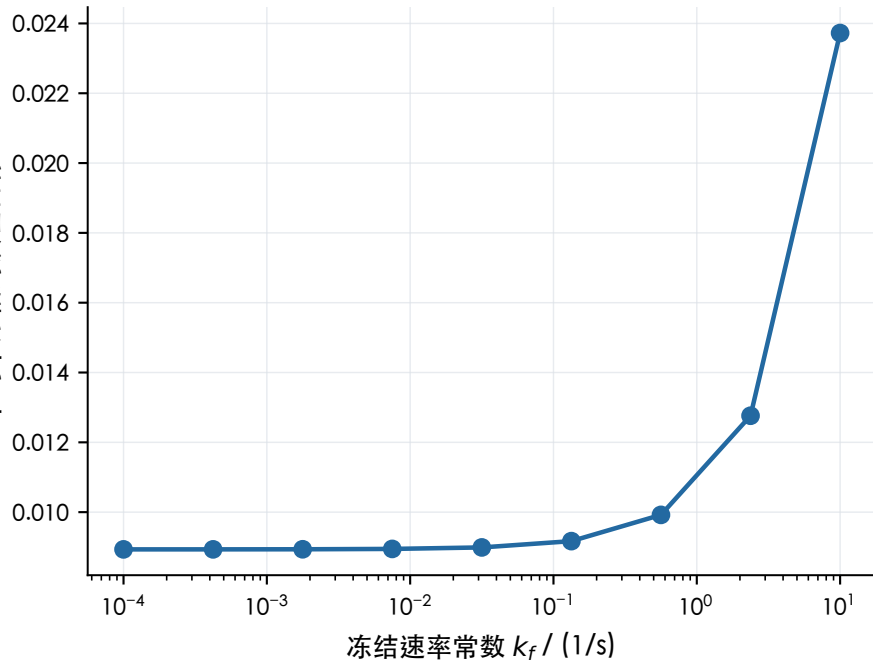
35 s 最大冰体积分数
