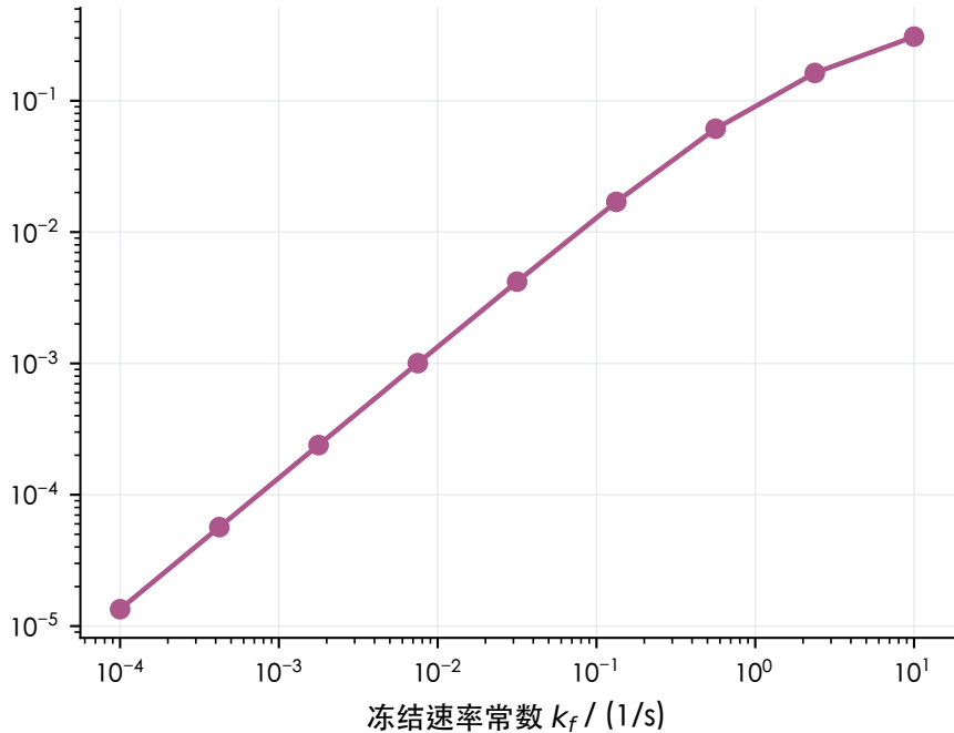
35 s 最大冰体积分数
