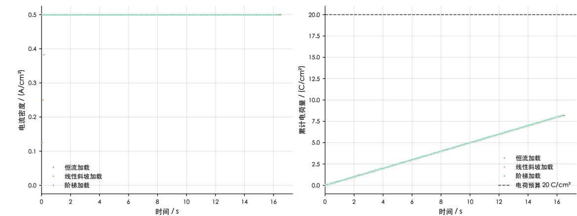
图 5-2 三种最优加载策略及累计电荷量随时间变化图 恒流加载与阶梯加载数据图重合
