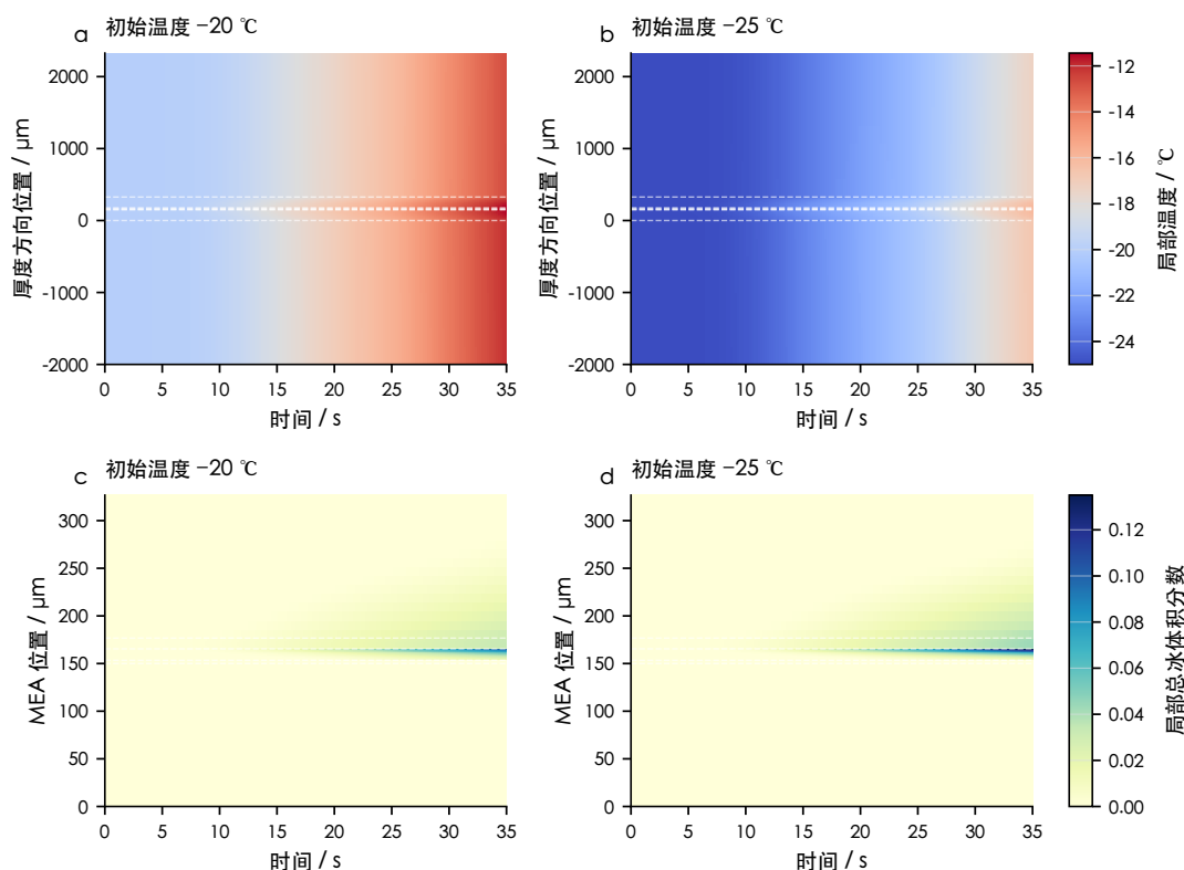
图 4-3 含双极板修订模型温度与结冰时空分布图
