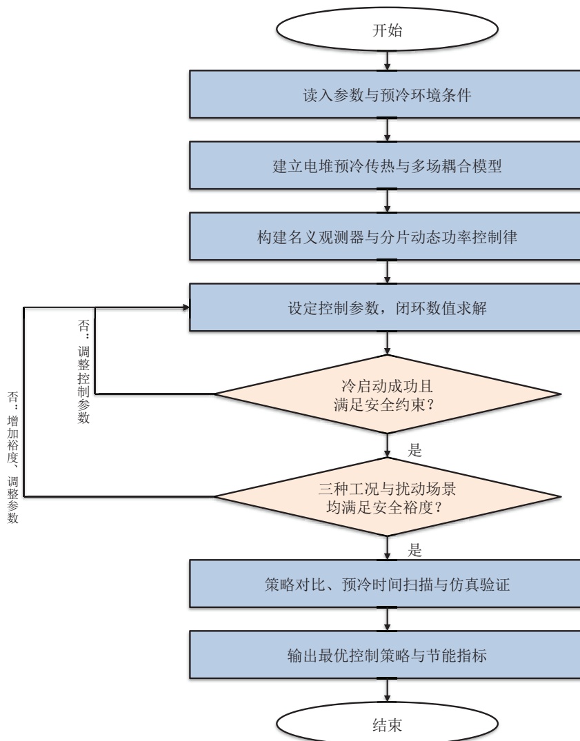
图 7-1 问题四：电堆动态辅助加热控制策略优化与预冷影响分析流程图
