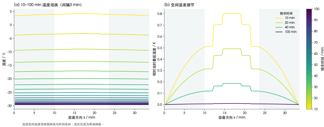
图 7-2 不同预冷时间下的整堆温度场及局部温差
