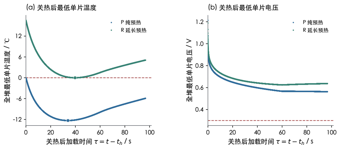
图 6-4 关热后温度回落与延长预热验证图
