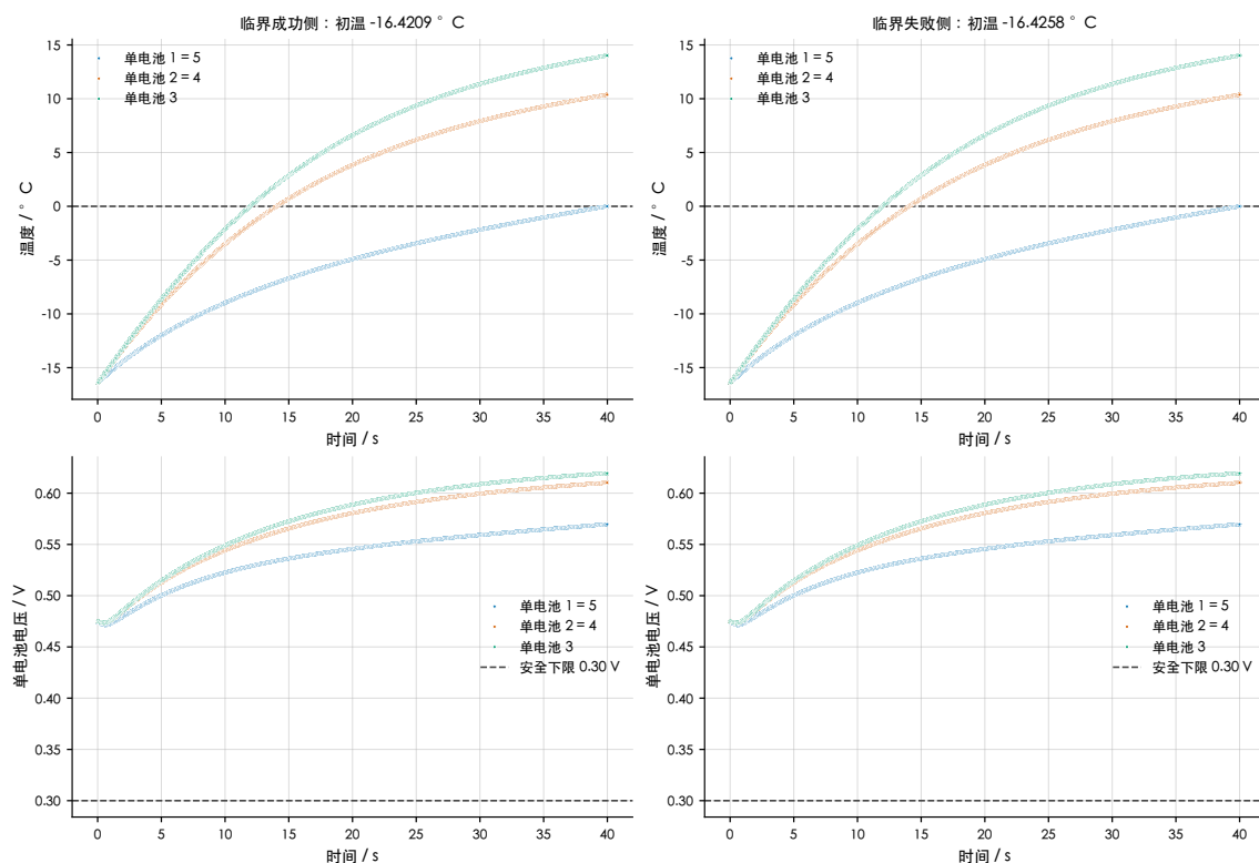
图 5-7 临界初温两侧各单电池温度与电压演化图
