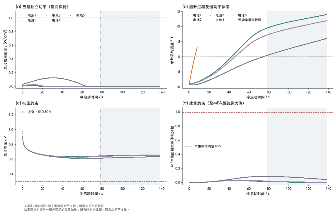
图 7-4 预冷 20 min 工况下推荐动态策略的功率与水热电状态演化
