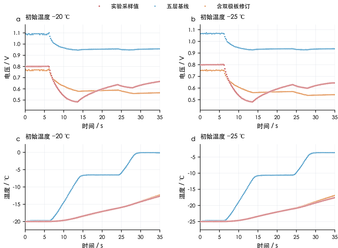
图 4-1 实验数据与五层基线与含双极板修订模型对比图
