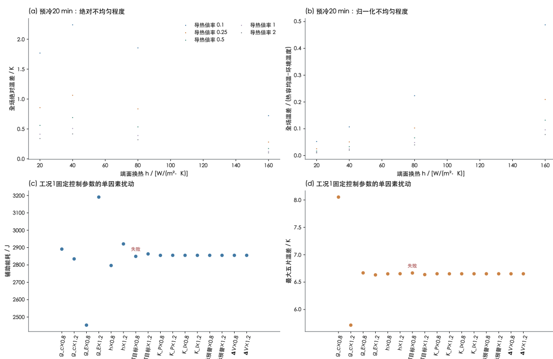
图 7-8 预冷传热参数与名义动态控制参数的敏感性
