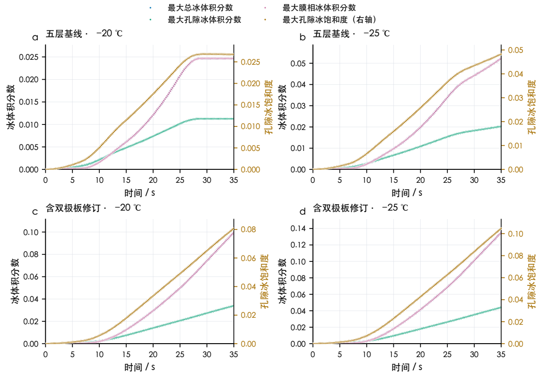
图 4-2 总冰孔隙冰膜相冰体积分数与孔隙冰饱和度图
