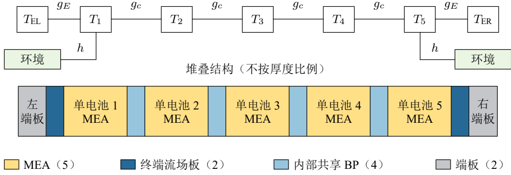
图 5-2 五片电堆结构及热耦合模型示意图
