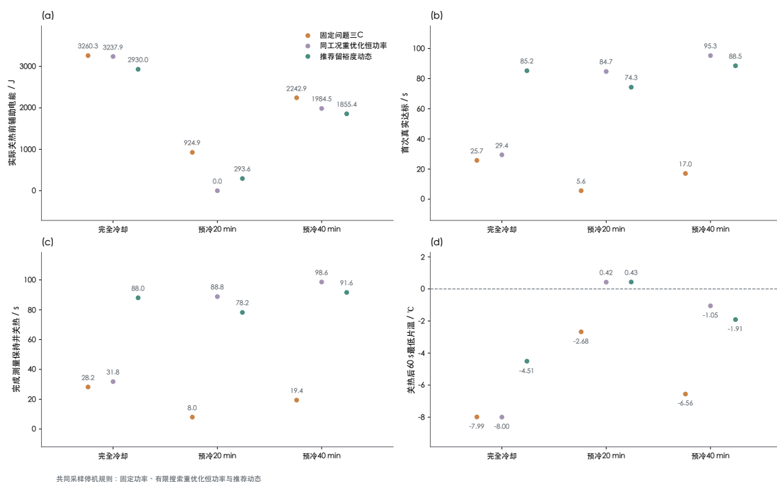
图 7-6 固定恒功率、同工况重新优化恒功率与推荐动态策略的比较
