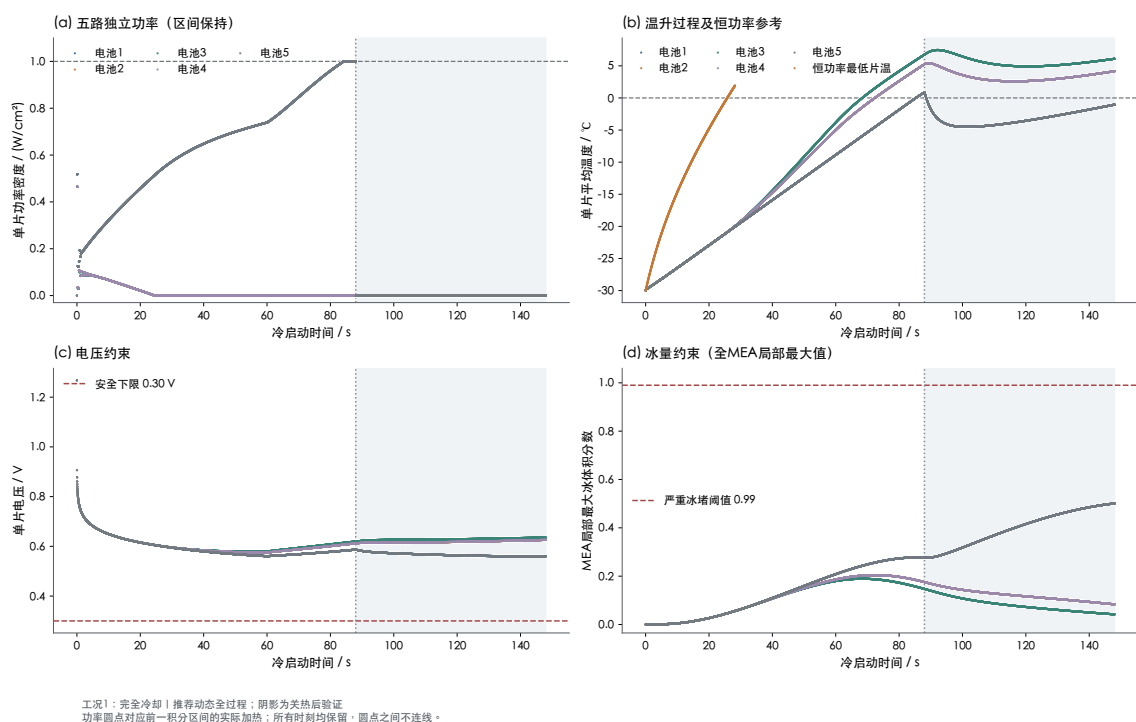
图 7-3 完全冷却工况下推荐动态策略的功率与水热电状态演化
