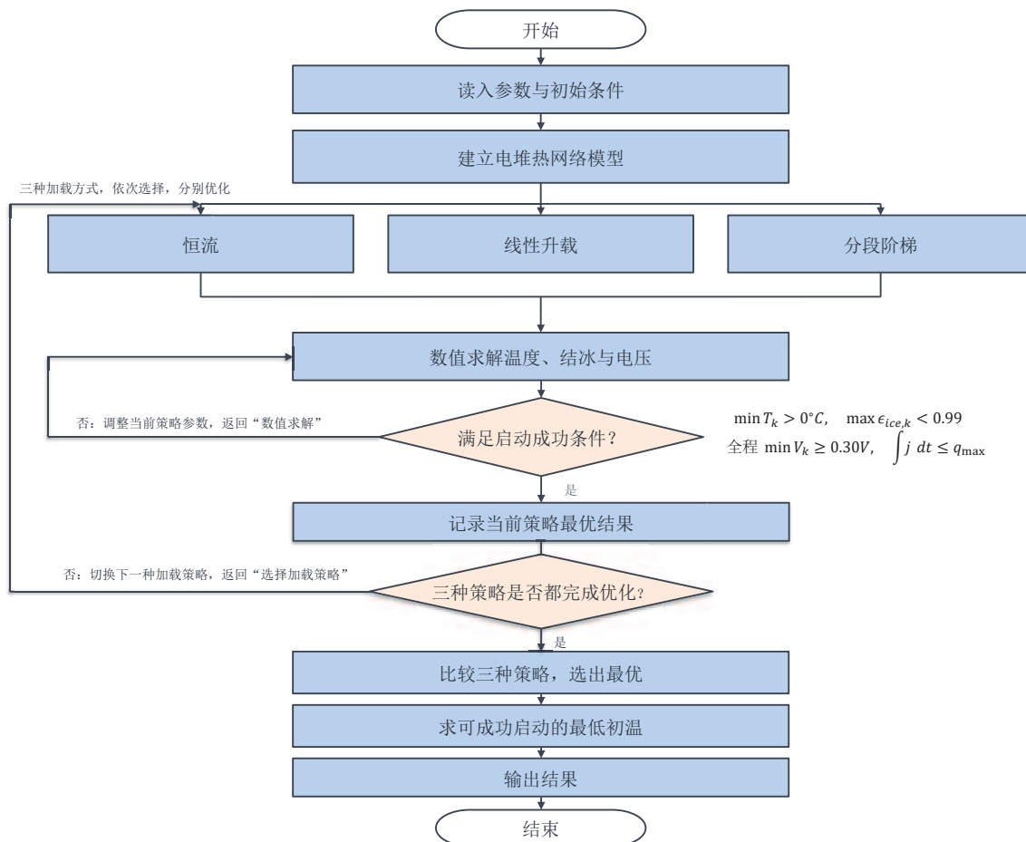
图 5-1 问题二：五片电堆瞬态自冷启动策略优化与最低初温搜索流程图
