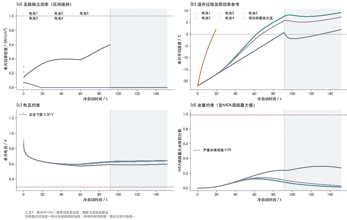
图 7-5 预冷 40 min 工况下推荐动态策略的功率与水热电状态演化
