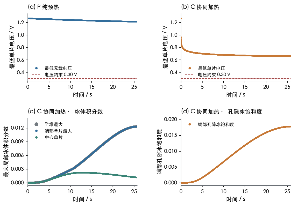
图 6-3 首次启动窗口内两策略电压与协同策略的局部结冰特征
