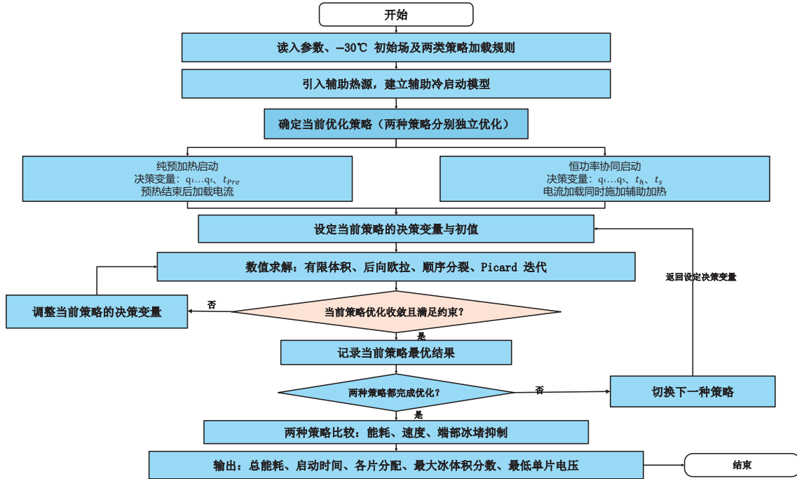
图 6-1 问题三：电堆辅助冷启动策略优化与对比流程图
