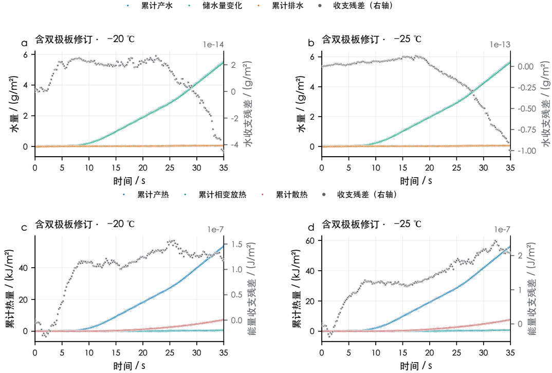
图 4-4 含双极板模型水量热量收支与守恒残差图
