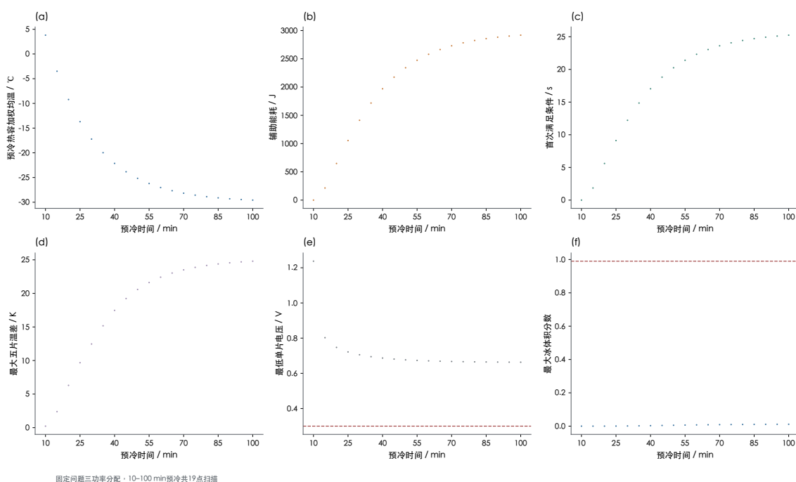
图 7-7 预冷时间对固定恒功率启动性能的影响
